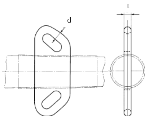
圖 10.2 附著於吊桿頭部之吊貨裝具
