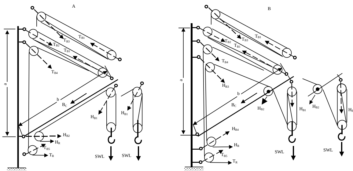
圖 A-2 重載起重設備之應力圖 (SWL 10 T及以上)
