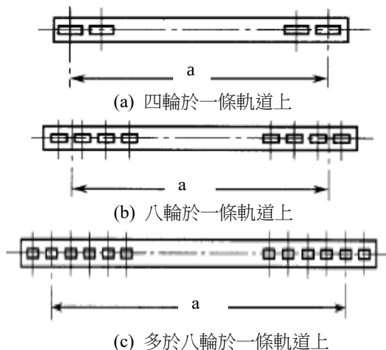
圖 9.1 有效輪基之量測
