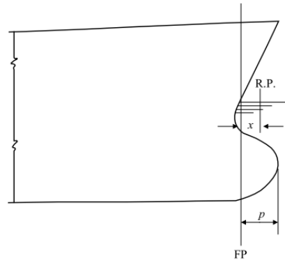
圖 III 2-17 具球型艏船舶之參考點
