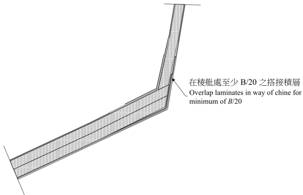
圖 III 2-35 稜艭或艙橫板-三明治構造
