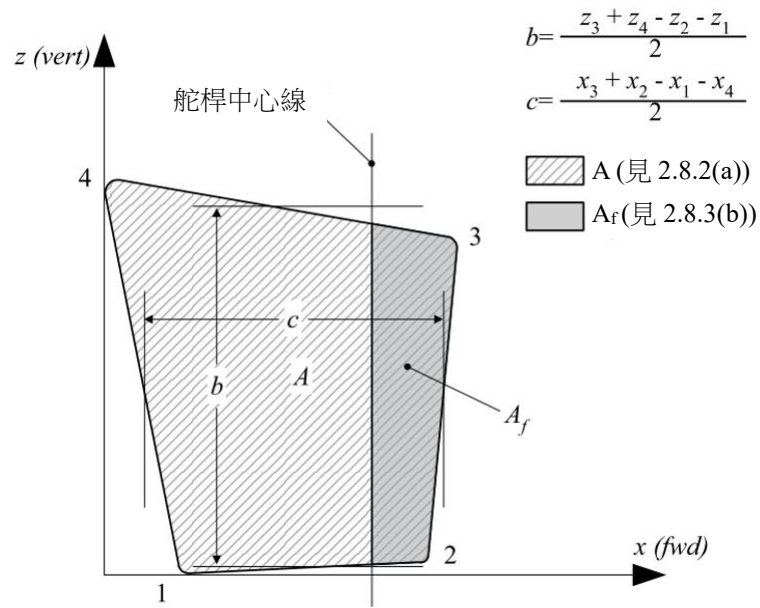
圖 III 2-39 完整舵葉
