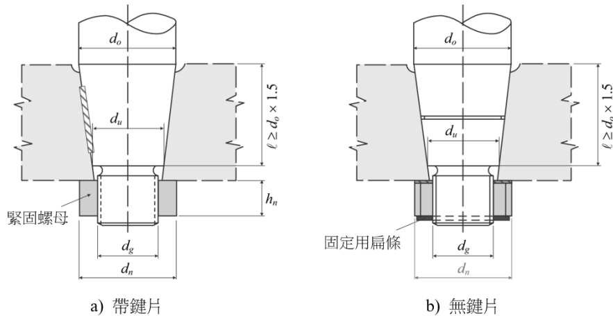
圖 III 2-43 錐形連結器
