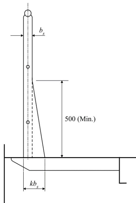
圖 III 2-56 欄杆支柱
