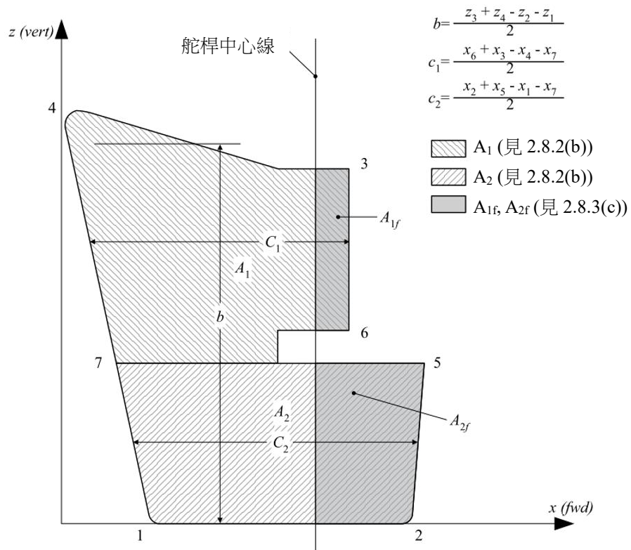
圖 III 2-40 缺角舵葉
