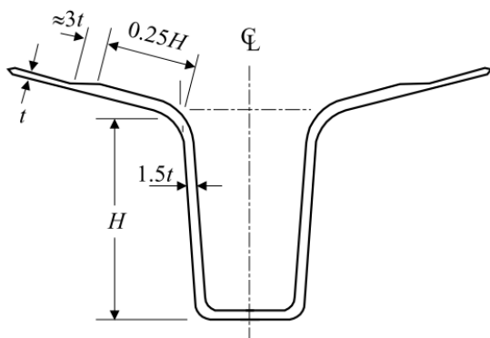
圖 III 2-33 垂直龍骨或艉鰭
