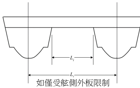
圖 III A2-2 跨甲板中心線剖面之典型幾何形狀
