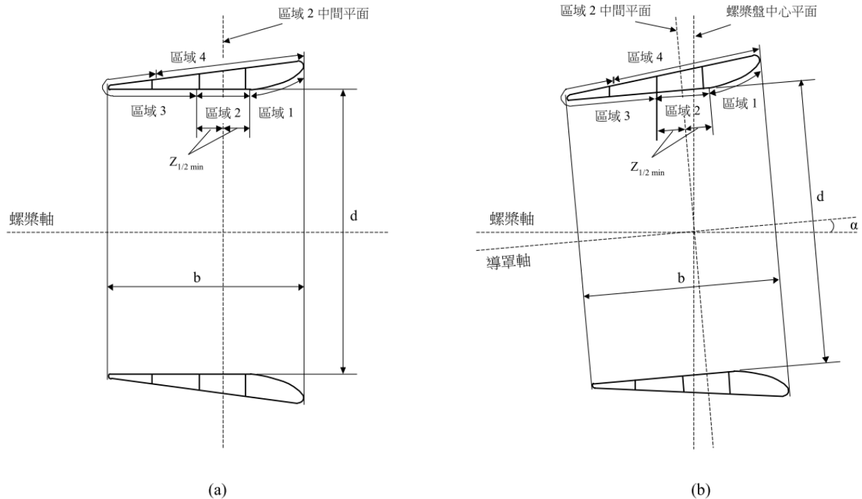
圖 III 2-38 導罩螺槳剖面圖
