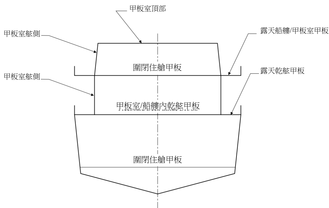
圖 III 2-6 甲板、船艙及甲板室壓力
