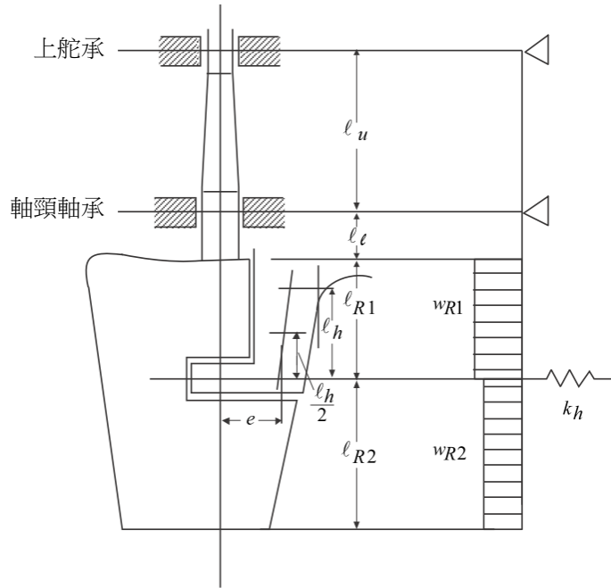
圖 III A1-3 以一舵針及半懸舵承架所支撐之舵
