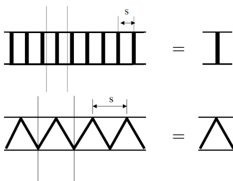
圖 III 2-12 擠壓板
