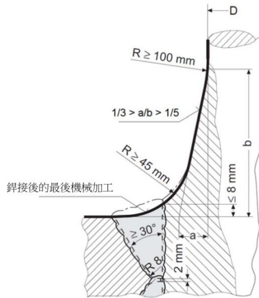
圖 III 2-42 舵桿與聯結器凸緣的銲接節點
