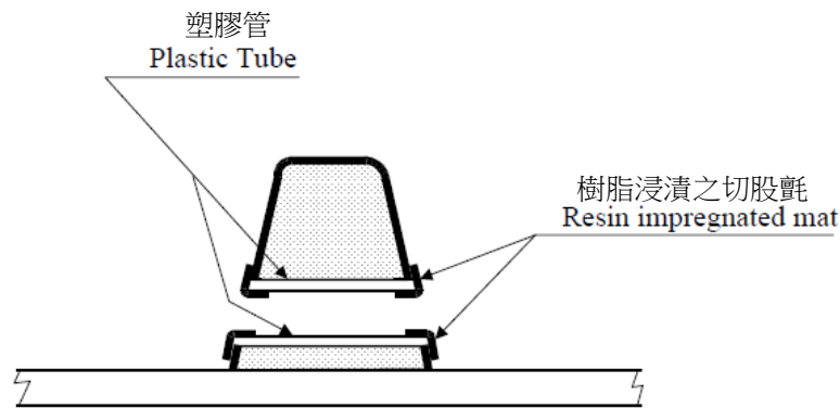
圖 III 2-20 貫穿過充滿發泡材空間之管路或開口
