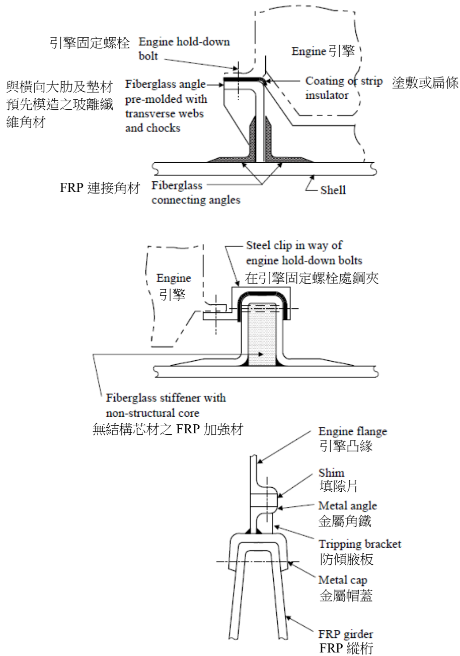
圖 III 2-25 引擎基座
