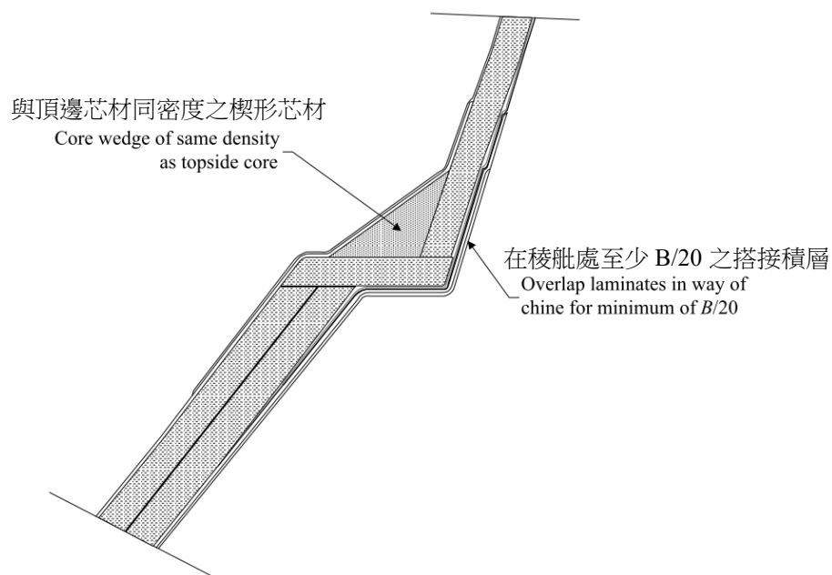
圖 III 2-36 階梯式稜艭-楔形發泡材選擇
