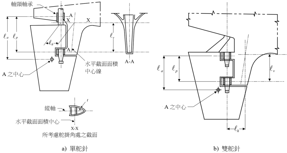
圖 III 2-44 舵掛角
