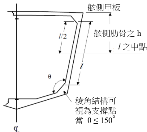
圖 III 2-13 橫向舷側肋骨
