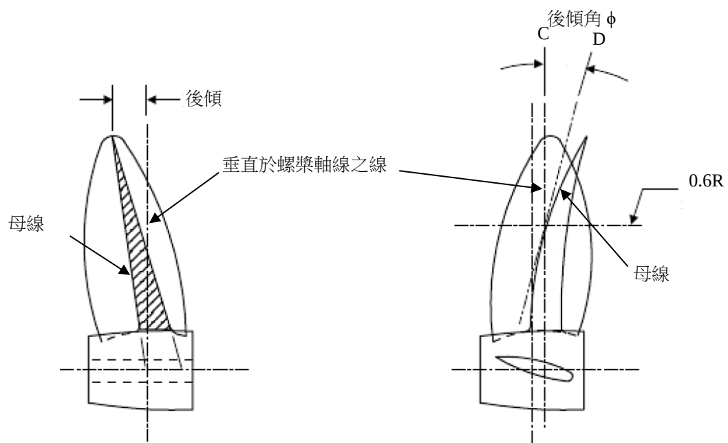
圖 IV 2-2 後傾與後傾角
