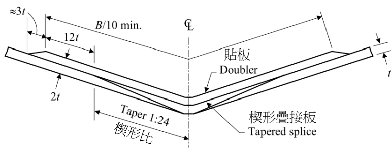
圖 III 2-32 分半積層船殼之平板龍骨
