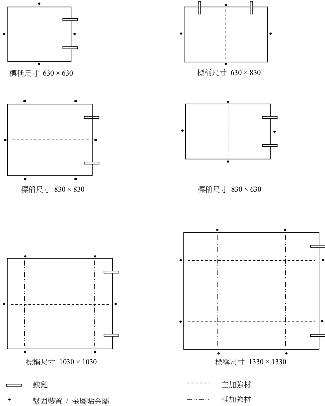
圖 III 2-50 加強材之布置
