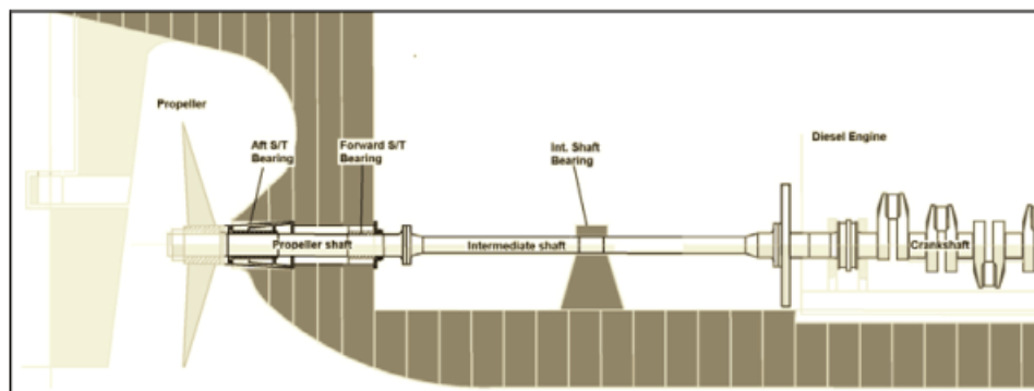
圖 I 2-1(a) 典型的軸系布置
