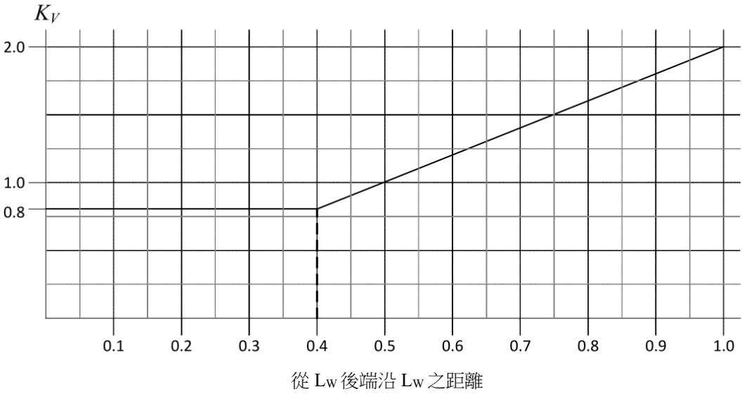
圖 III 2-8 垂直加速度分配係數 K_V
