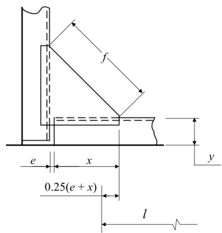
圖 III 1-5 腋板
