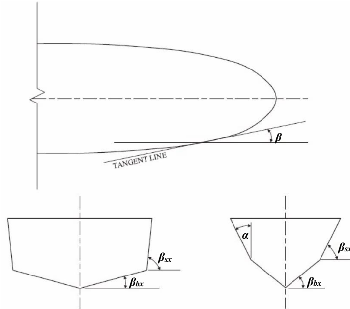
圖 III 2-5 橫斜高、舷緣外傾及進入角
