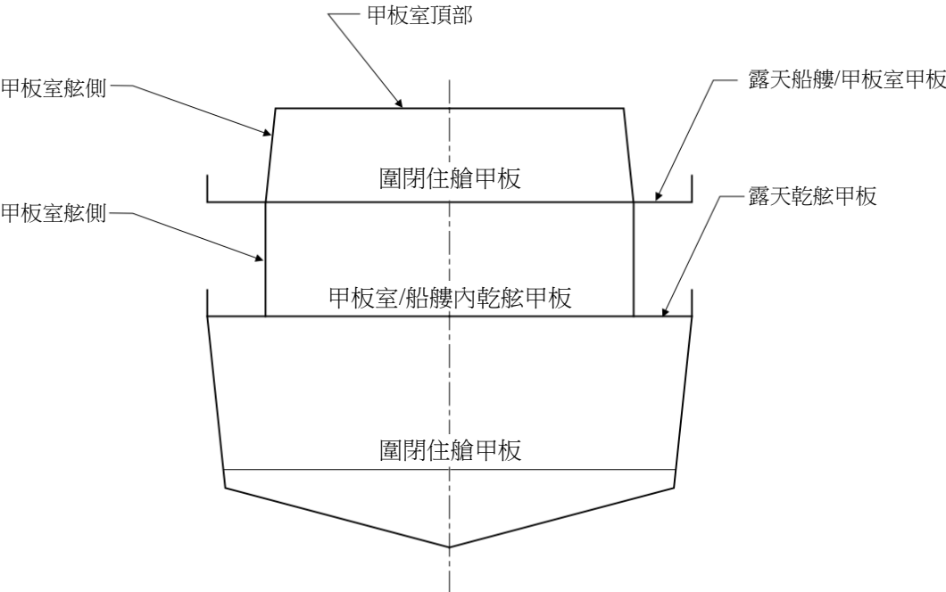
圖 III 2-6 甲板、船艙及甲板室壓力
