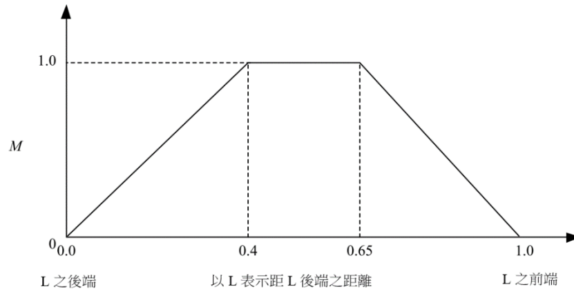
圖 III 2-2 分佈係數 M
