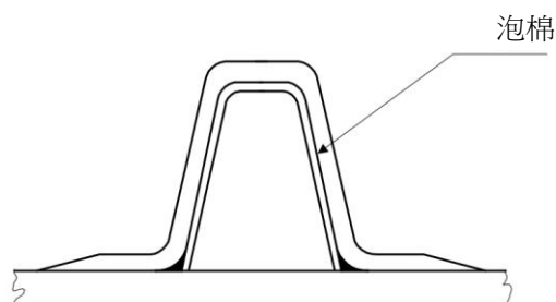
圖 III 2-22 預先模造FRP型材
