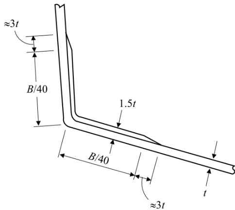
圖 III 2-34 稜舳或艏橫板-單板構造
