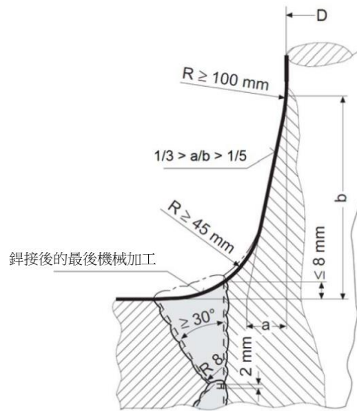
圖 III 2-42 舵桿與聯結器凸緣的銲接節點
