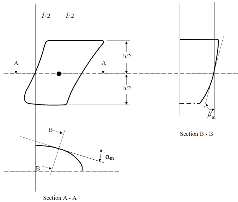
圖 III 2-53 \alpha_m 及 \beta_m 之定義
