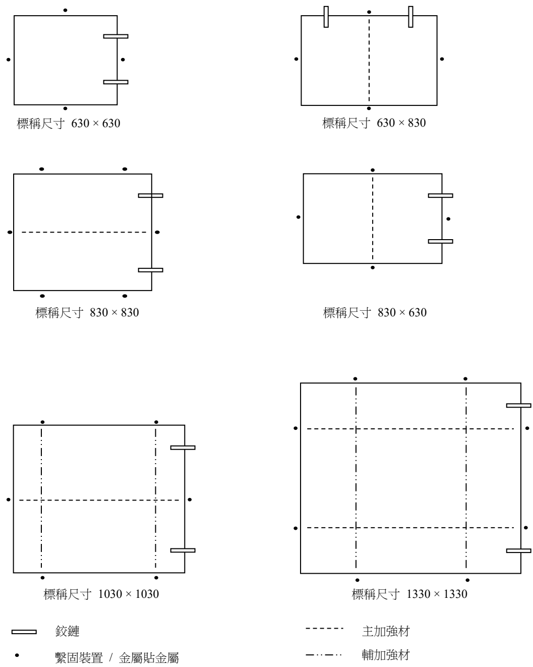
圖 III 2-50 加強材之佈置
