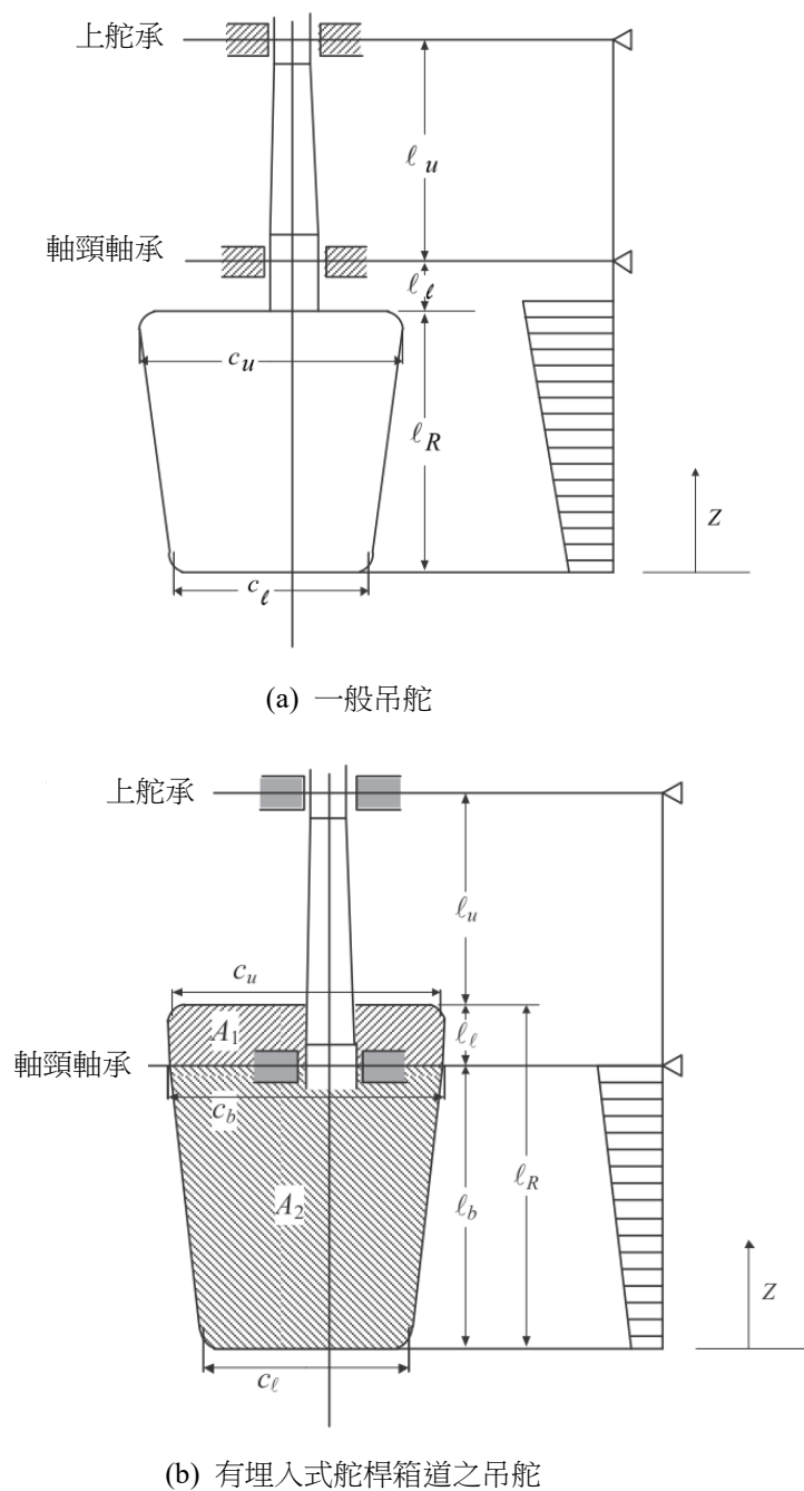
圖 III A1-1 吊舵
