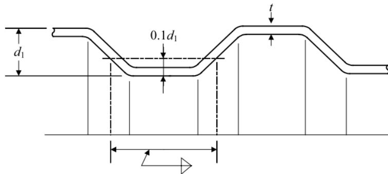
圖 III 2-16 波形船壁端部連接
