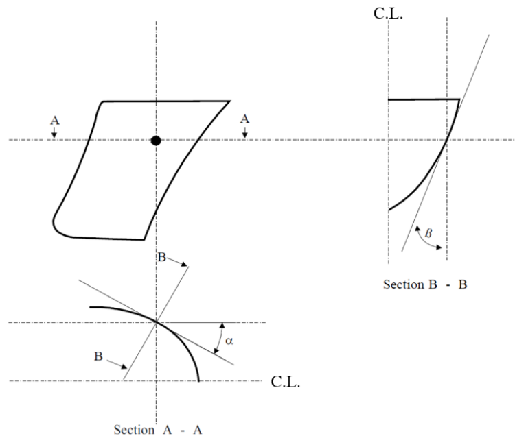
圖 III 2-52 進入角及舷緣外傾角
