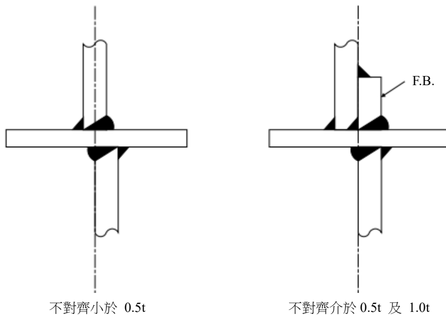
圖 II 2-2 不對齊之修理
