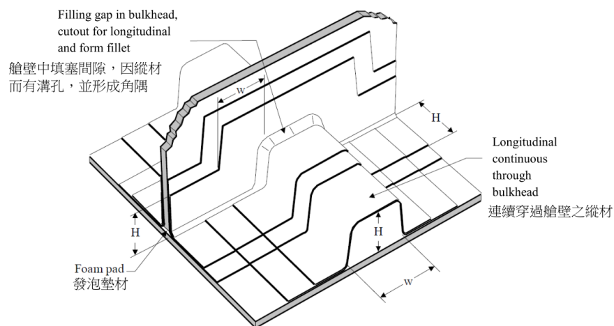
圖 III 2-24 縱向材與橫向材之連接
