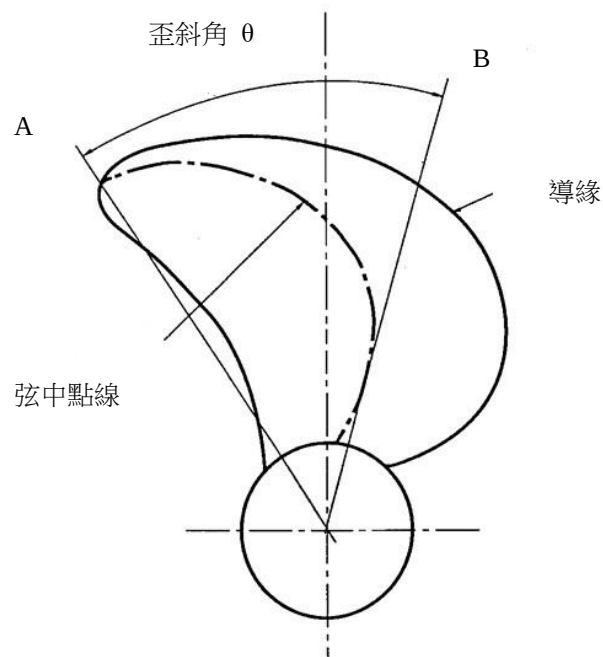
圖 IV 2-1 最大歪斜角
