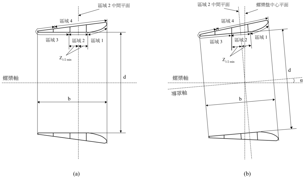
圖 III 2-38 導罩螺槳剖面圖
