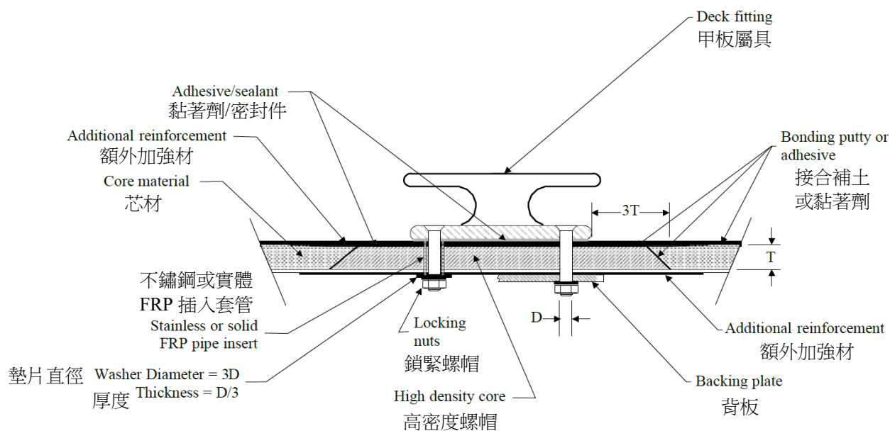
圖 III 2-26 甲板裝具
