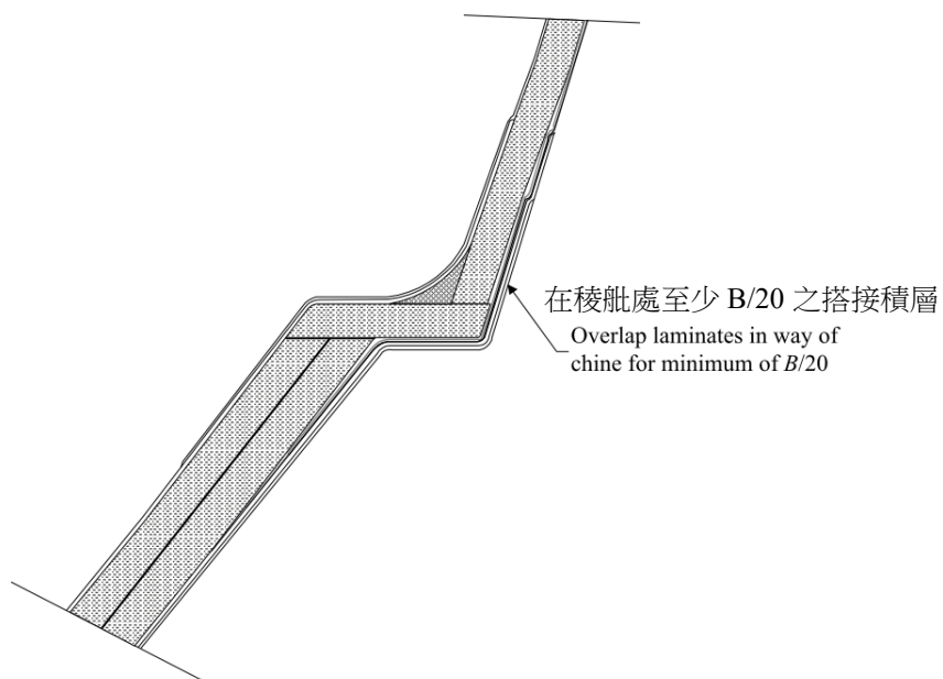
圖 III 2-37 階梯式稜觥-補土半徑
