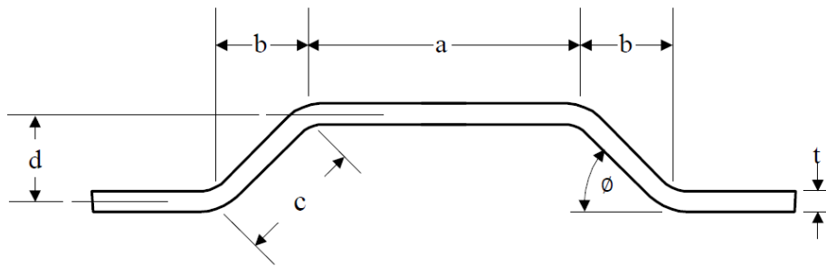
圖 III 2-15 波形船壁
