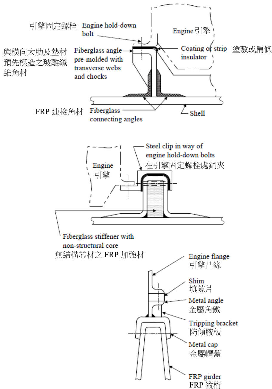
圖 III 2-25 引擎基座
