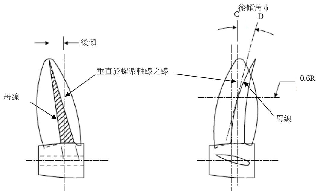
圖 IV 2-2 後傾與後傾角
