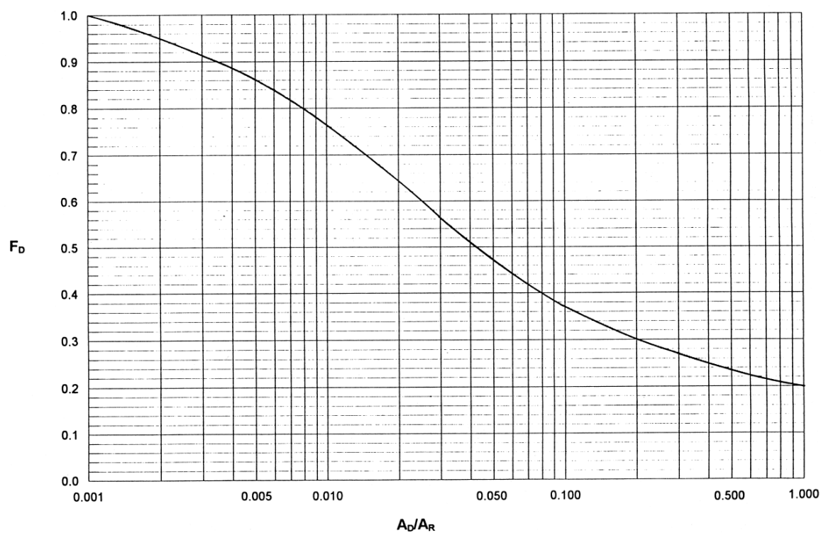
圖 III 2-7 設計面積係數 F_D
