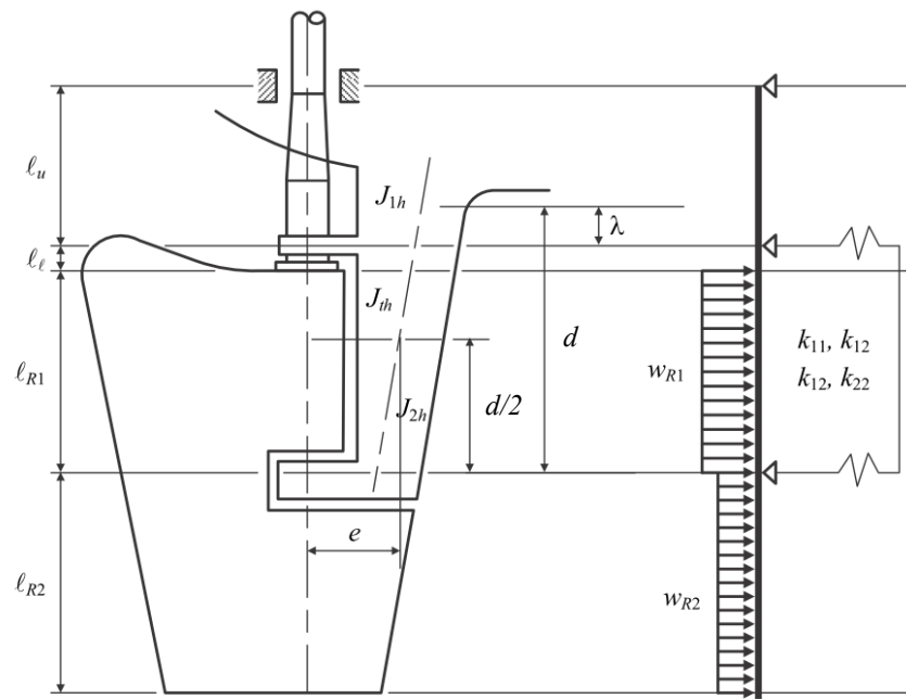
圖 III A1-4 設有兩個舵針(支架)的半懸舵承架所支撐之舵
