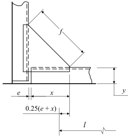
圖 III 1-5 腋板
