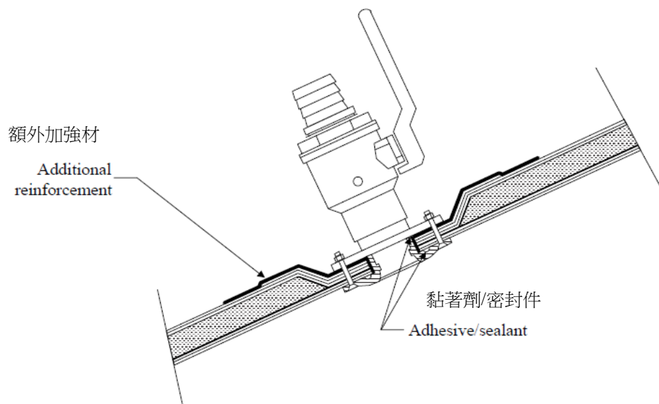
圖 III 2-27 穿過船殼貫穿件-實體積層
