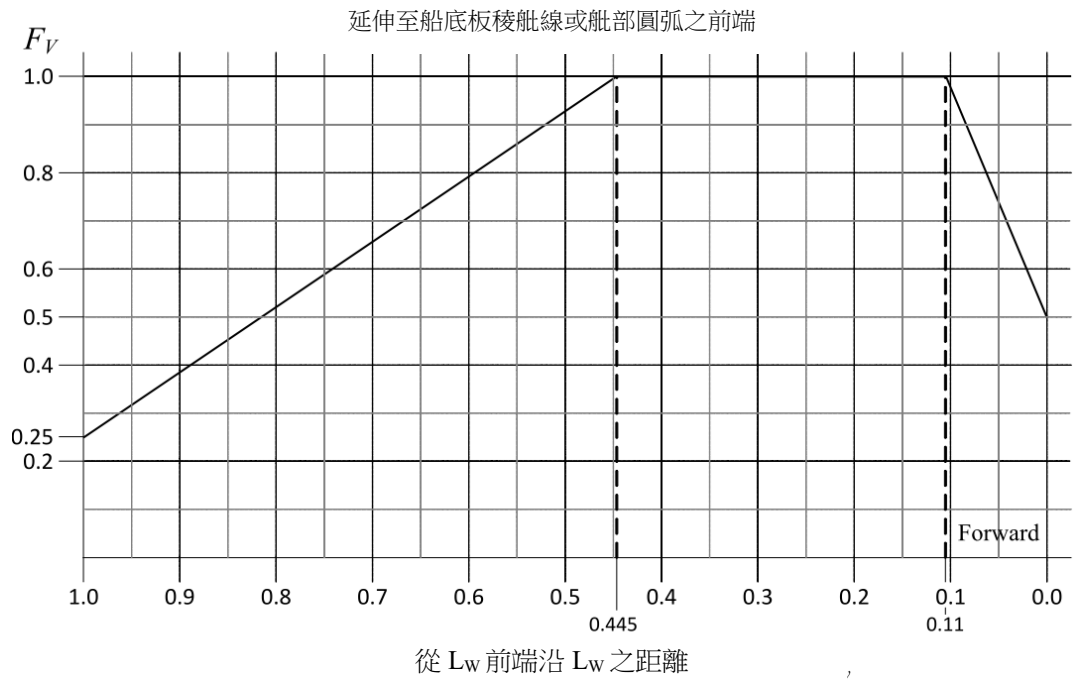
圖 III 2-9 垂直加速度分配係數 F_v
