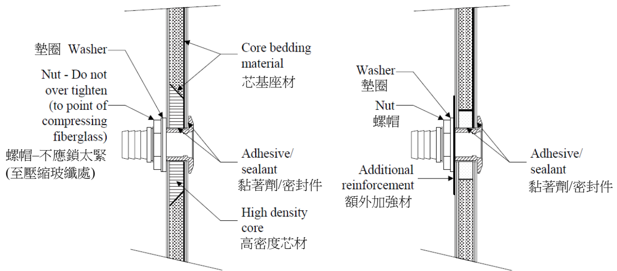
圖 III 2-28 穿過船殼貫穿件-三明治積層
