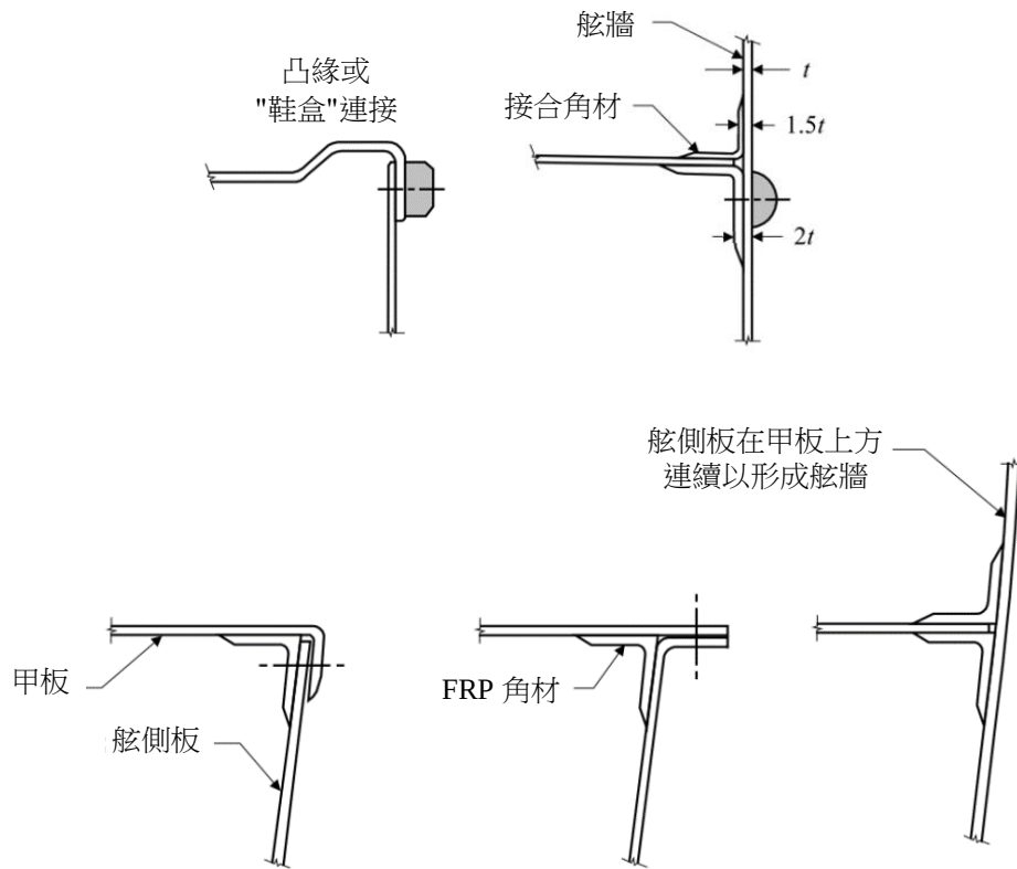
圖 III 2-30 甲板對船殼露天連接之示例
