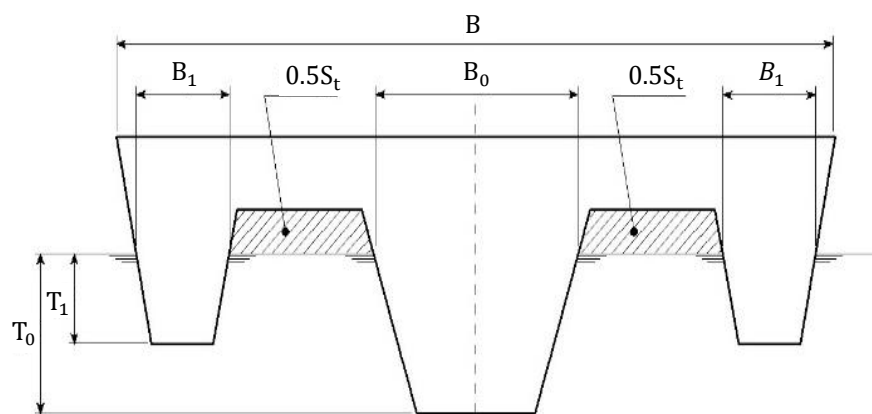
圖 III 5-2 具有隧道區的多體船
