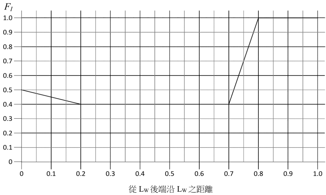
圖 III 2-10 濕面積分配係數 F_l
