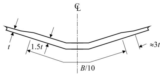
圖 III 2-31 一體積層船殼之平板龍骨
