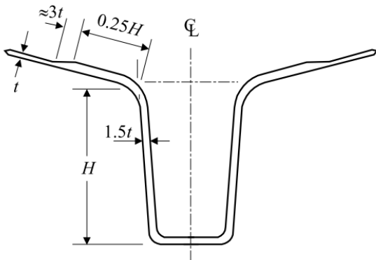
圖 III 2-33 垂直龍骨或舵鰭
