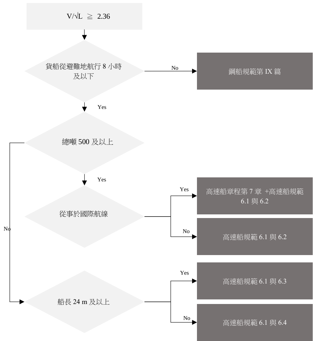
圖 IV 6-1 船舶個別類型適用規範
