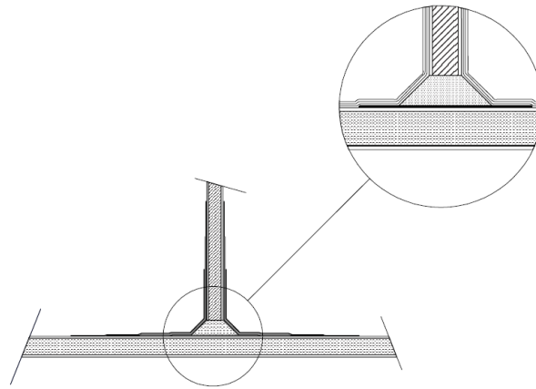
圖 III 2-29 FRP構件之邊界角材
