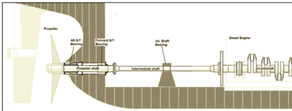
圖 I 2-1(a) 典型的軸系佈置
