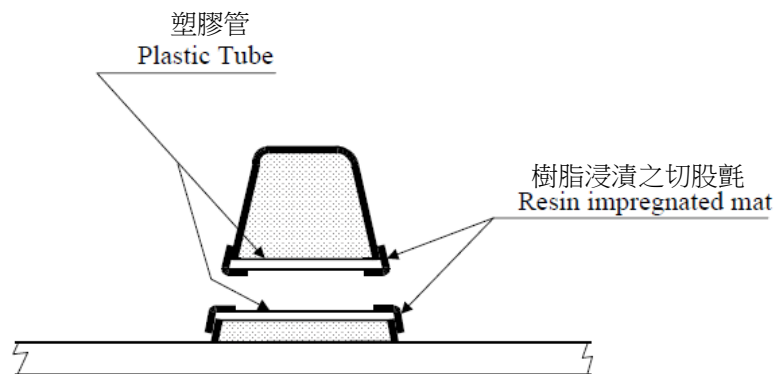
圖 III 2-20 貫穿過充滿發泡材空間之管路或開口
