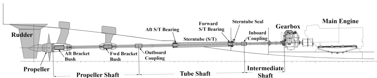
圖 I 2-1(b) 典型的水潤滑軸系
