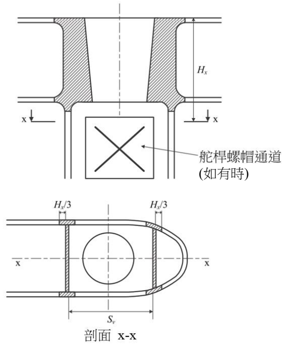
圖 III 2-49 舵葉與舵桿承座連接處剖面
