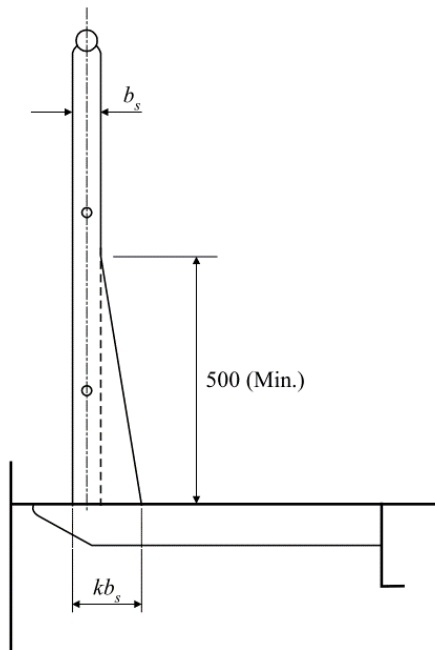
圖 III 2-56 欄杆支柱
