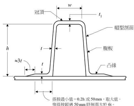
圖 III 2-21 加強材之比例
