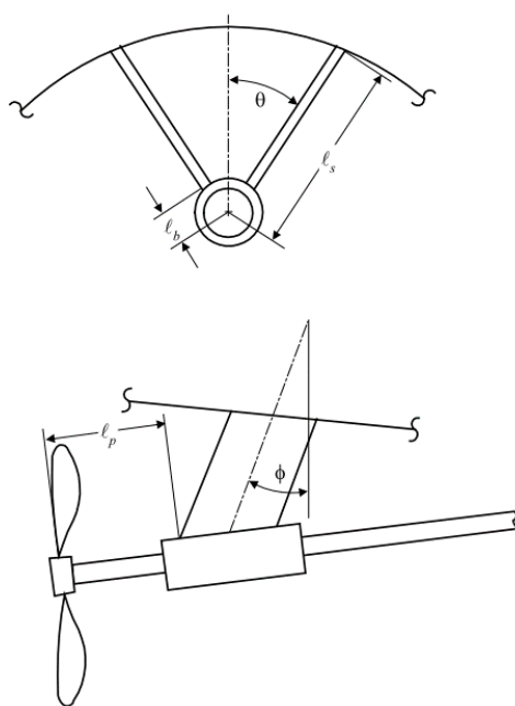
圖 III A3-1 軸架尺寸
