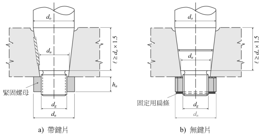
圖 III 2-43 錐形連結器
