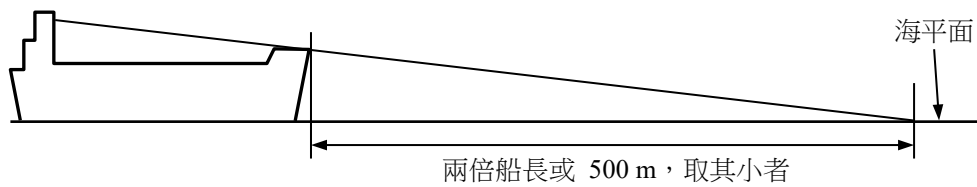
圖 III 6-1 指揮位置之海平面視界
