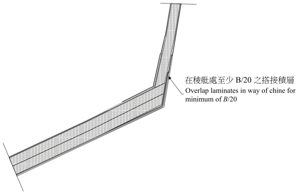
圖 III 2-35 稜艚或艚橫板-三明治構造
