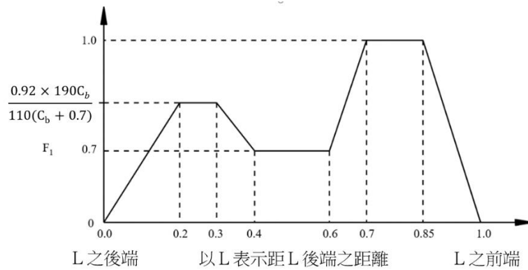
圖 III 2-3 分佈係數 F_1
