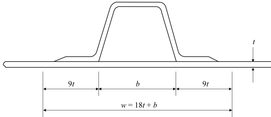
圖 III 1-6 FRP 板材之有效寬度
