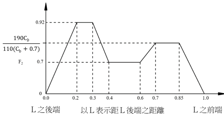
圖 III 2-4 分佈係數 F_2
