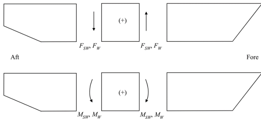
圖 III 2-1 正負符號
