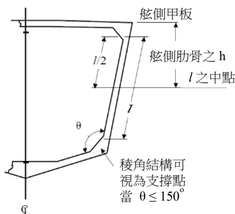
圖 III 2-13 橫向舷側肋骨
