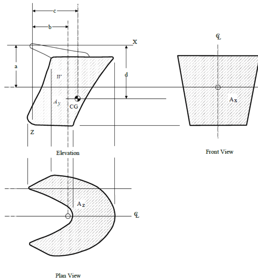
圖 III 2-54 掀起式艙門
