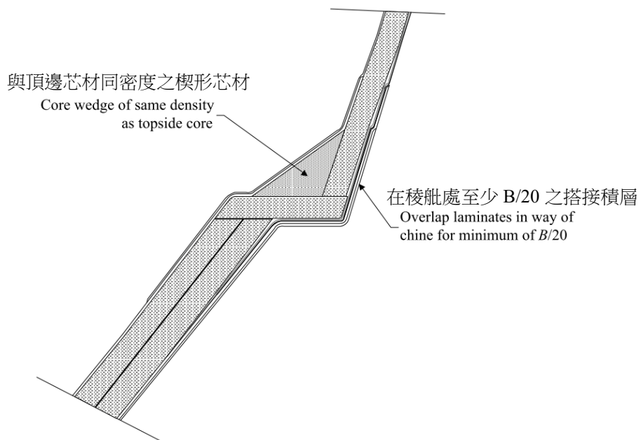
圖 III 2-36 階梯式稜艚-楔形發泡材選擇
