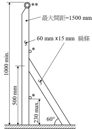
標準支柱、欄杆及支架寸法 (每 3 根支柱應提供支架)
