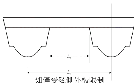
圖 III A2-2 跨甲板中心線剖面之典型幾何形狀
