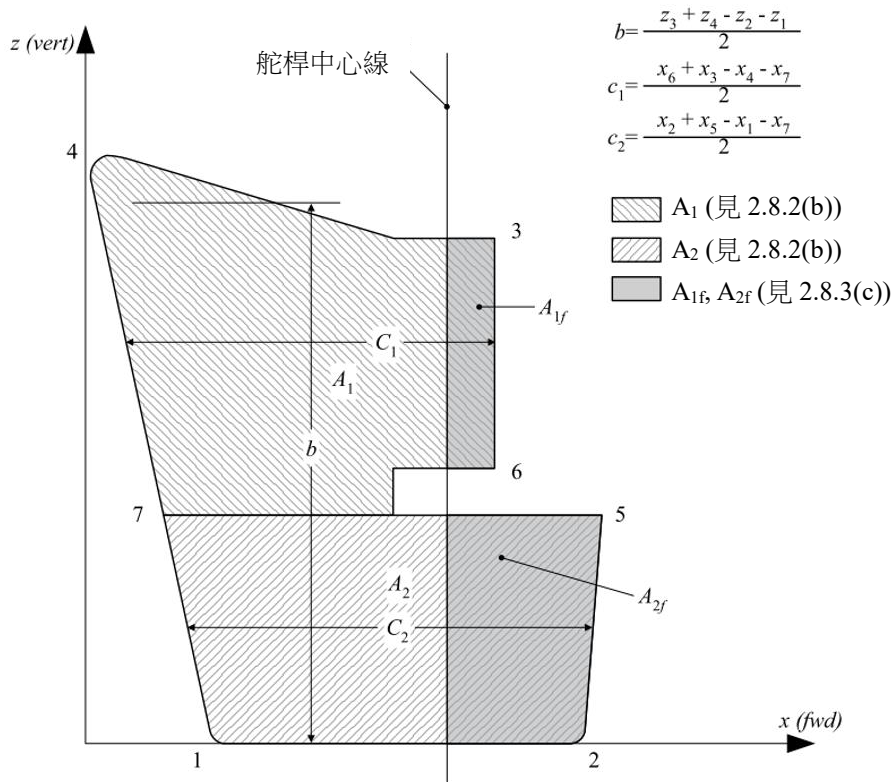
圖 III 2-40 缺角舵葉
