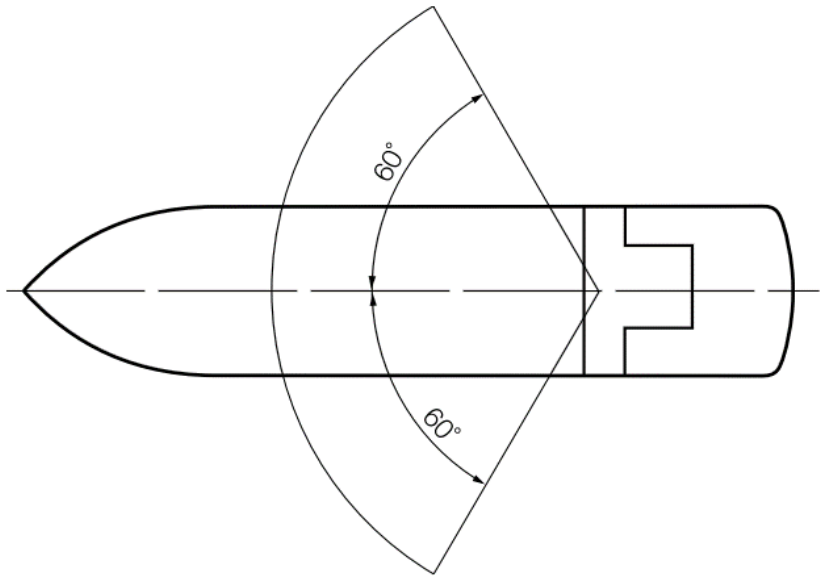
圖 III 6-4 主操舵位置之水平視野
