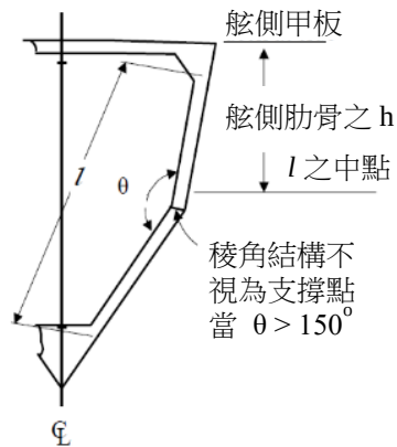
圖 III 2-14 橫向舷側肋骨
