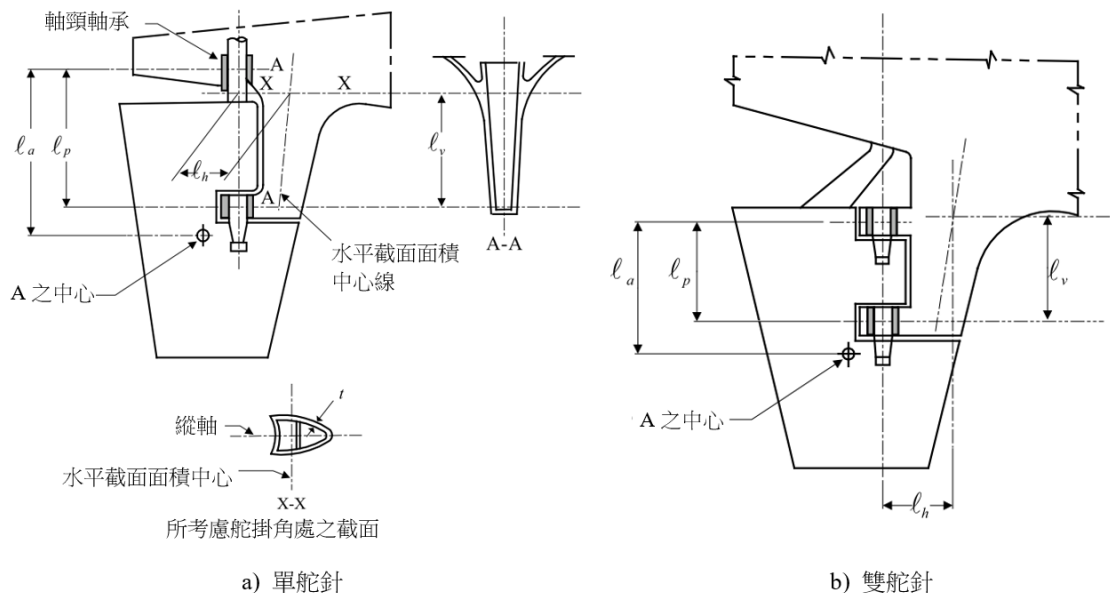
圖 III 2-44 舵掛角
