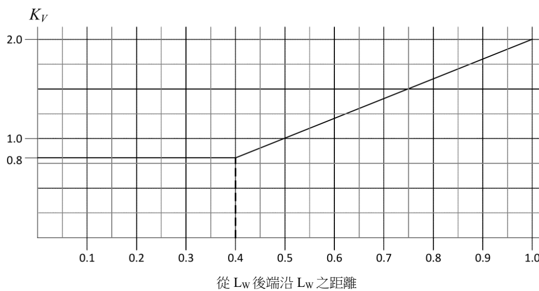
圖 III 2-8 垂直加速度分配係數 K_V
