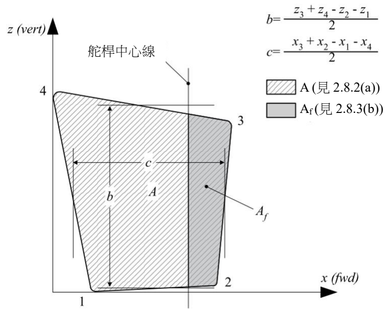
圖 III 2-39 完整舵葉
