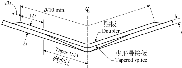
圖 III 2-32 分半積層船殼之平板龍骨
