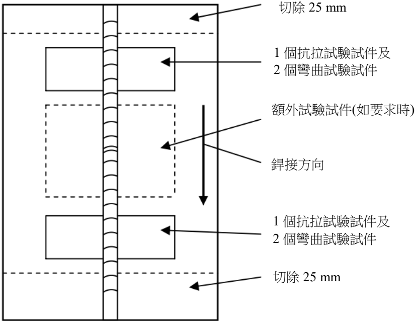
圖 II 2-7 板材對接銲試件之位置
