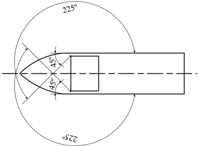
圖 III 6-3 每一駕駛橋艙兩翼之水平視野
