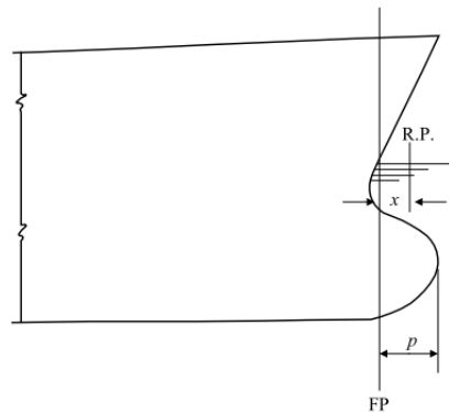
圖 III 2-17 具球型艙船舶之參考點
