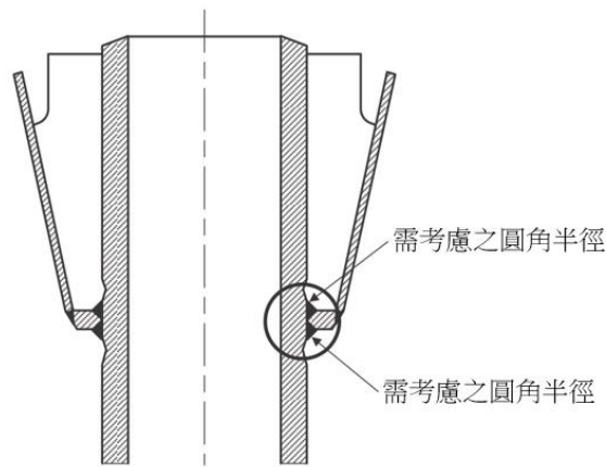
圖 III 2-41 凸肩圓角半徑
