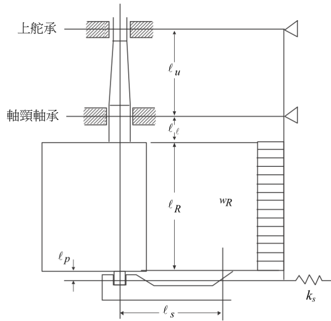
圖 III A1-2 舵跟材所支撐之舵
