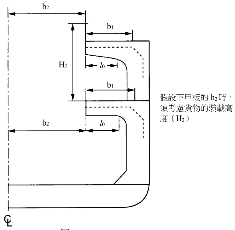
圖 II 6-3 l_0 、 b_1 、 b_2 及 H_2 的測量
