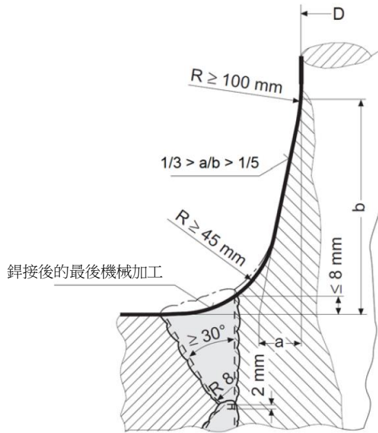
圖 II 24-6 舵桿與聯結器凸緣的銲接接頭
