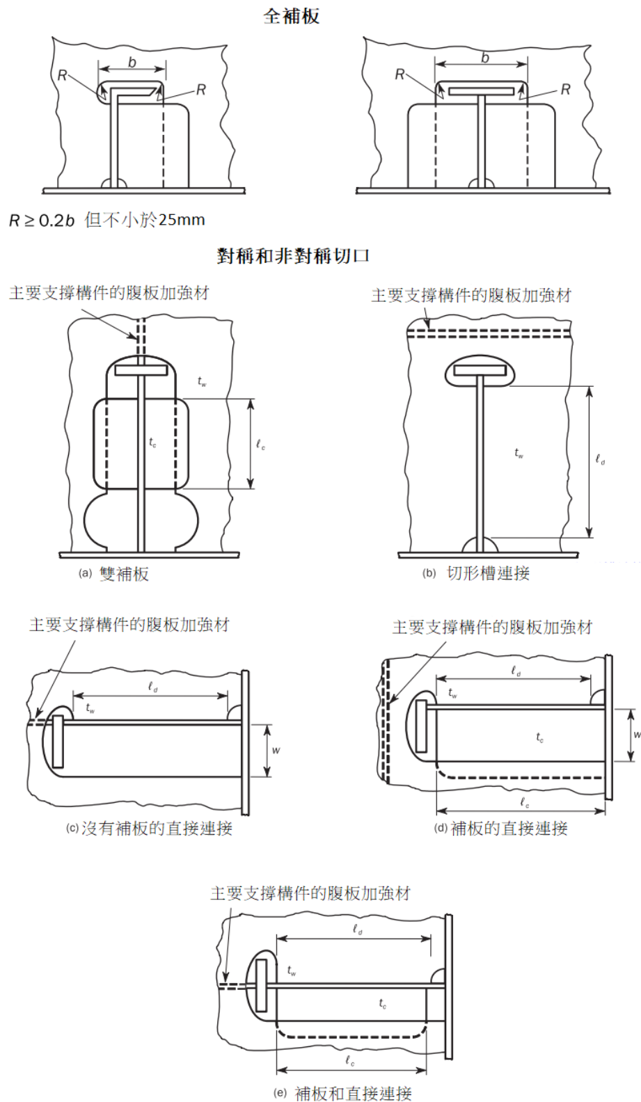
圖 II 1-6 切口和連接
