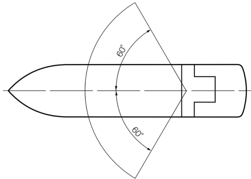
圖 III 6-4 主操舵位置之水平視野
