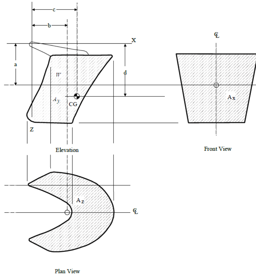
圖 III 2-54 掀起式艙門
