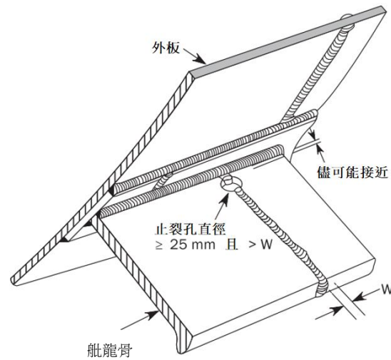
圖 II 1-8 舳龍骨構造
