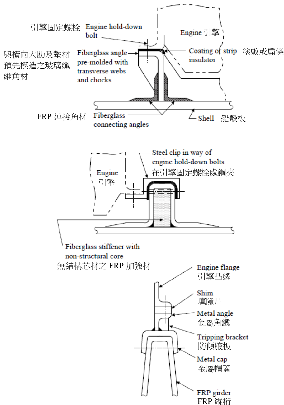
圖 III 2-25 引擎基座
