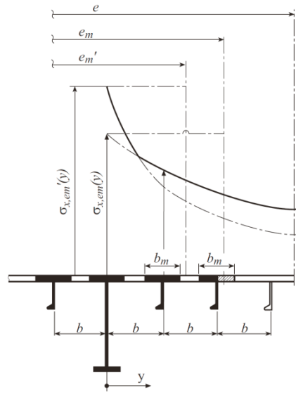
圖 II 17-4 平行主支撐構件腹板之加強
