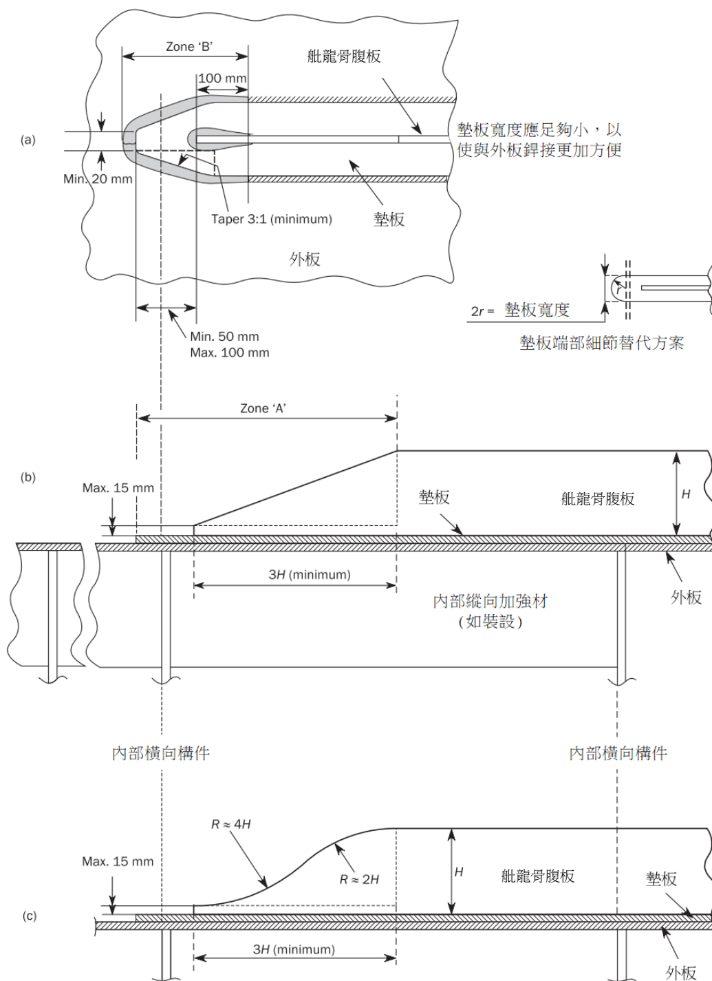
圖 II 1-9 舳龍骨端部設計
