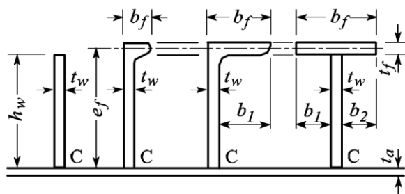
圖 II 17-6 加強材尺寸
