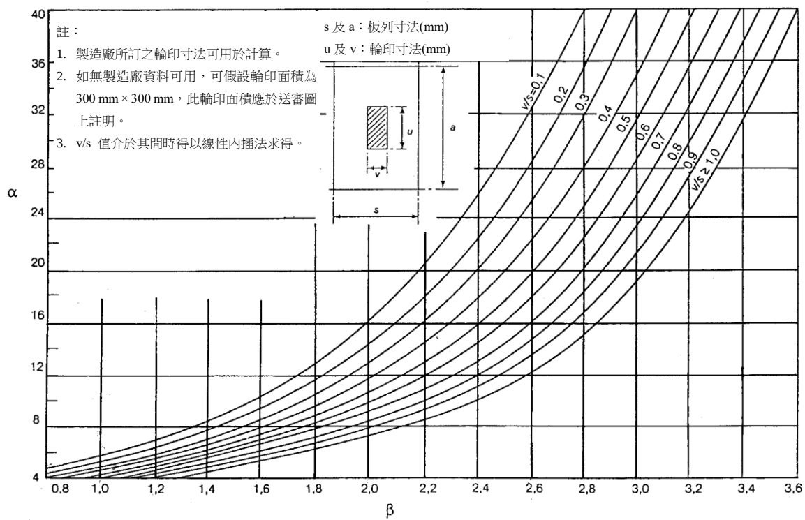
圖 II 12A-1 輪印曲線
