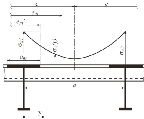
圖 II 17-5 垂直主支撐構件腹板之加強
