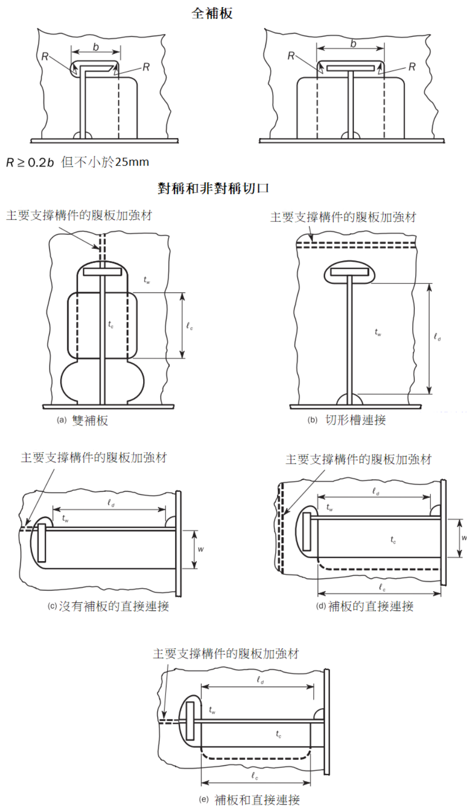
圖 II 1-6 切口和連接
