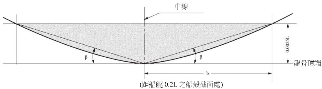
圖 II 8-1 b 之測量
