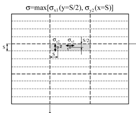
圖 II 17-1 艙口蓋板正應力之決定
