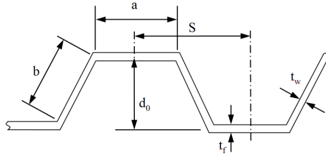
圖 II 14-2 S 的量測
