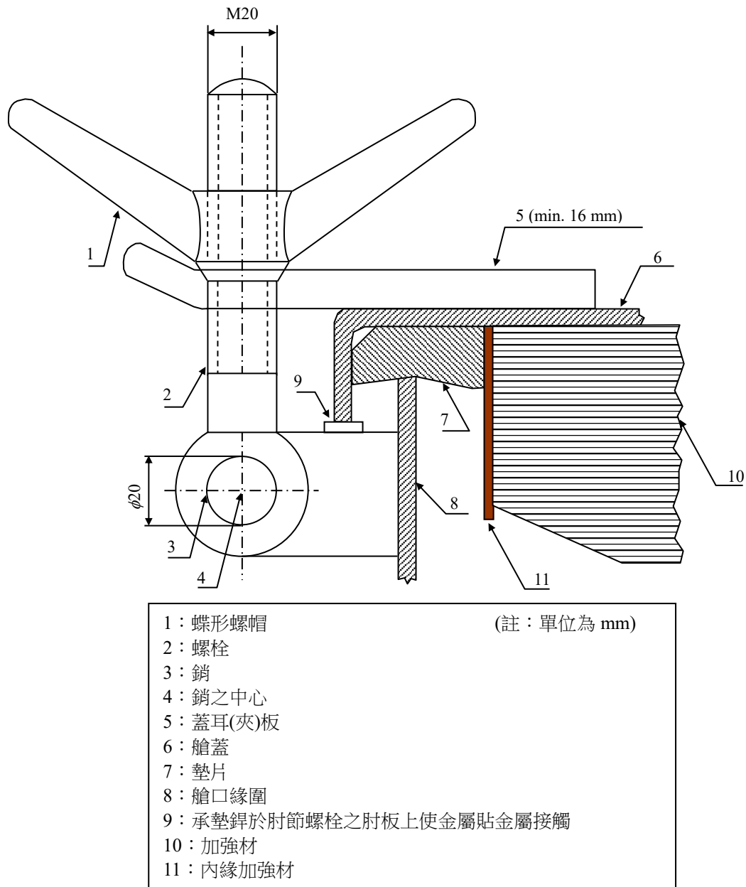
圖 II 27-2 主繫固法之例
