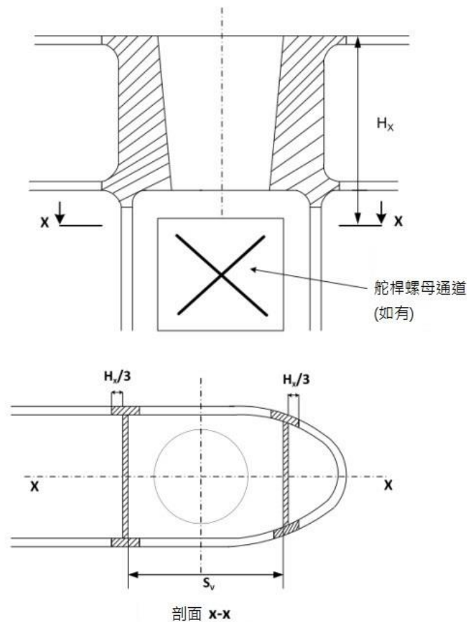
圖 II 24-5 舵葉與舵桿承座連接處剖面
