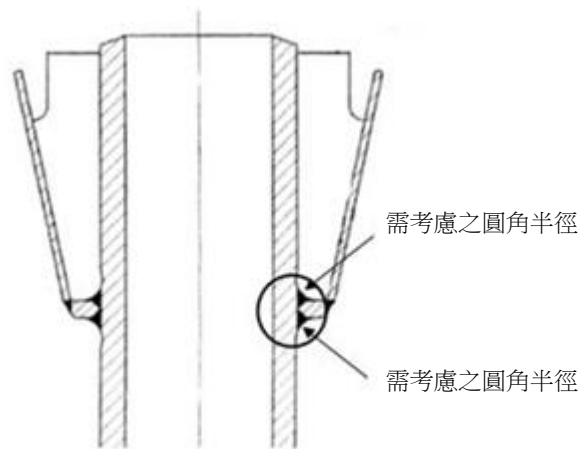
圖 II 24-9 圓角肩部半徑
