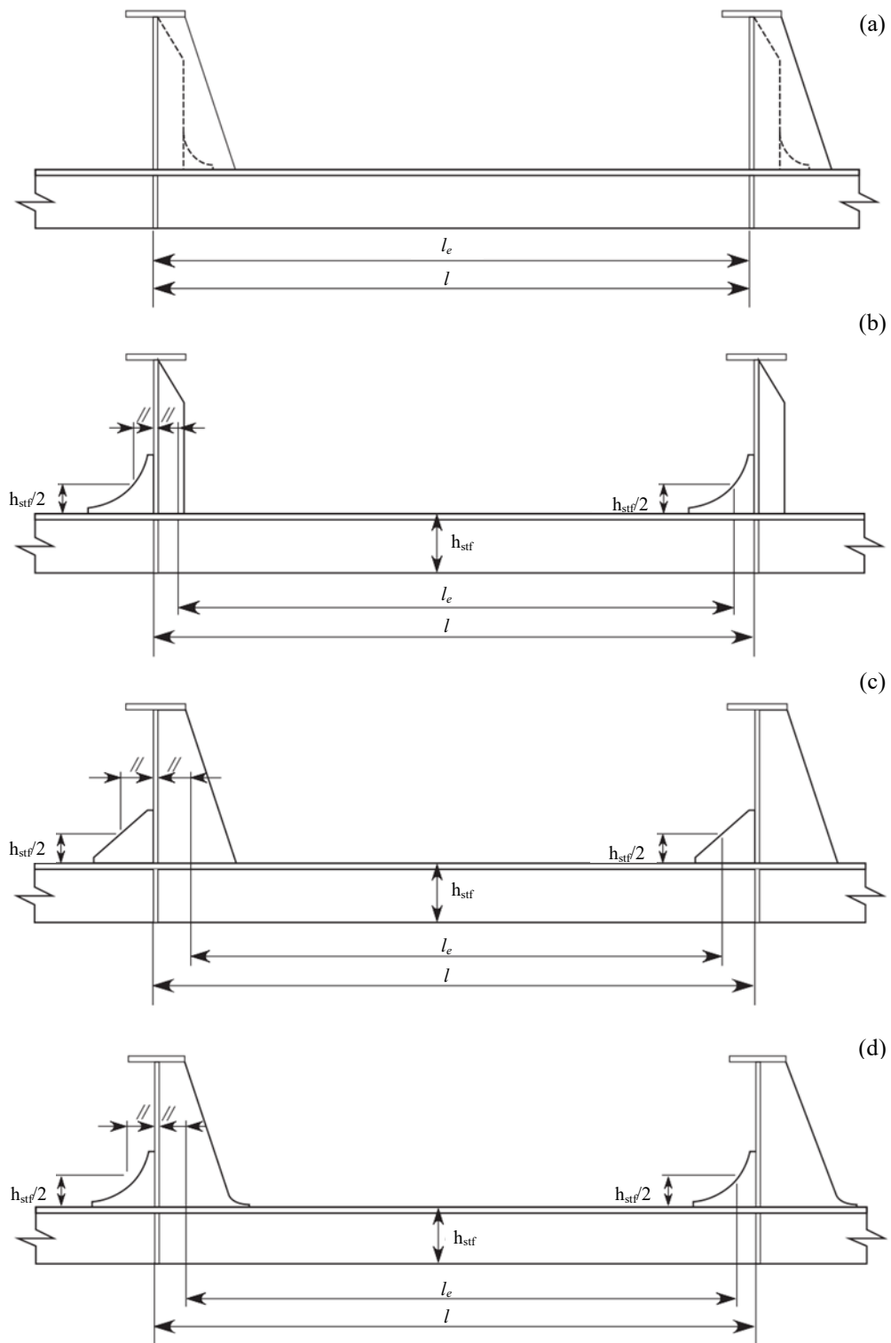
圖 II 1-2 由腹板加強材支撐之加強材的有效彎曲跨距(單殼構造)
