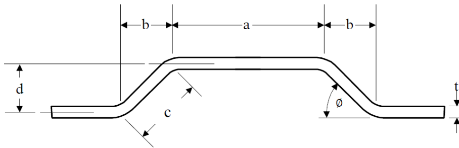
圖 III 2-15 波形船壁
