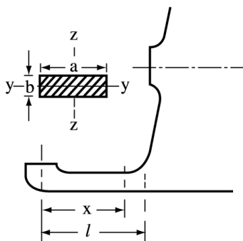
圖 II 2-2 舵跟材
