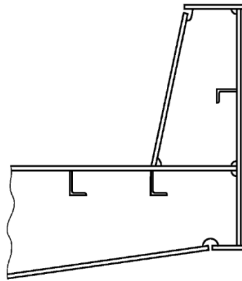
圖 II 17-8 緣圍板延伸範例
