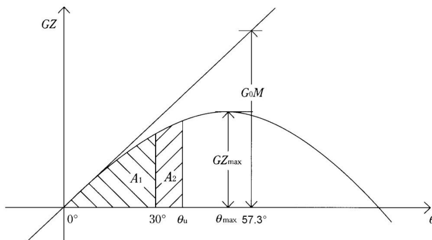
圖 II 30-1 穩度曲線(一般穩度準則)
