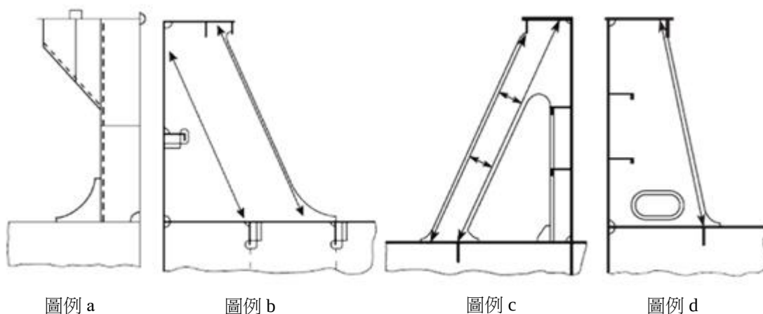
圖 II 17-7 緣圍支撐範例
