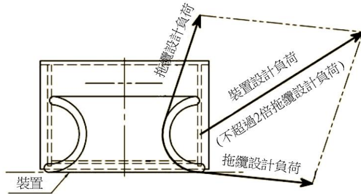
圖 II 25-1 設計負荷
