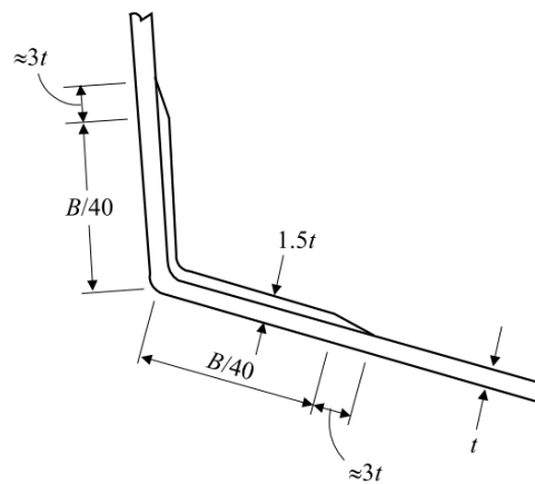
圖 III 2-34 稜艚或舵橫板-單板構造
