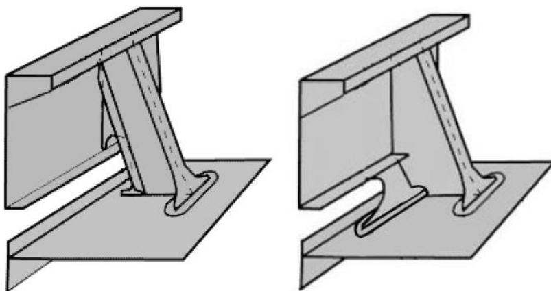
圖 II 13-1 腋板型式(左) 以及 角牽型式(右)
