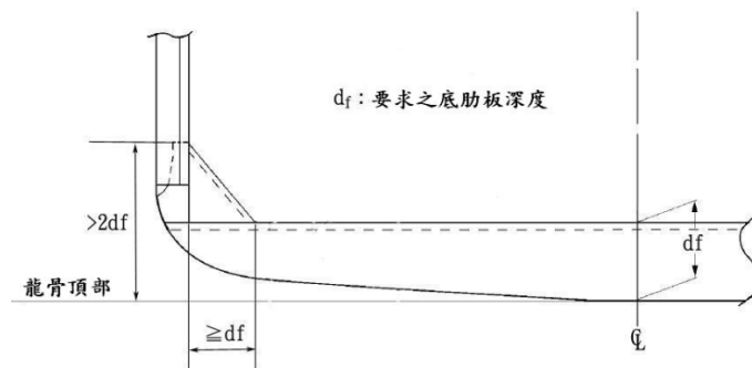
圖 II 4-1 側肋骨腋板
