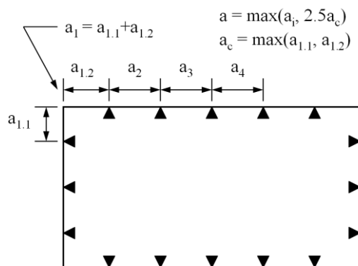
圖 II 17-2 鎖固裝置之間的距離，沿艙口蓋外圍量取
