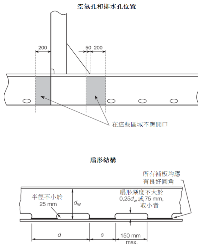
圖 II 1-7 空氣孔、排水孔及扇形孔
