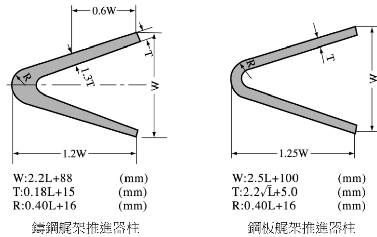
圖 II 2-1 推進器柱之標準
