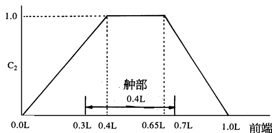
圖 II 3-2 C 2 係數
