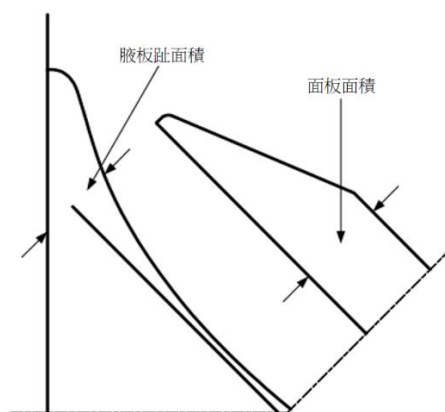
圖 II 1-5 腋板趾部結構
