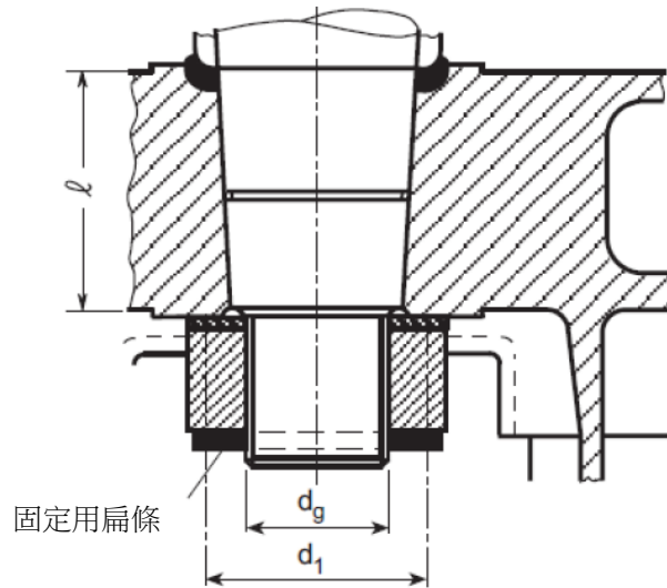
圖 II 24-8 無鍵片錐形聯結器
