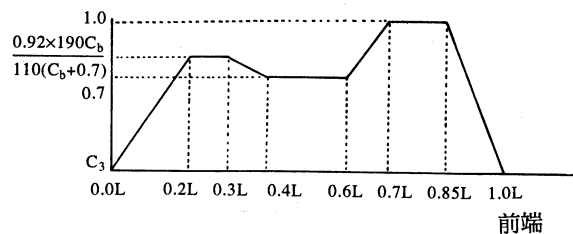
圖 II 3-4 分佈係數 C_3
