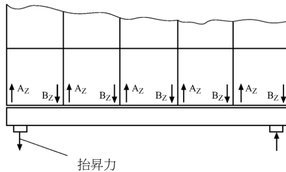
圖 II 17-9 艙口蓋的抬昇力
