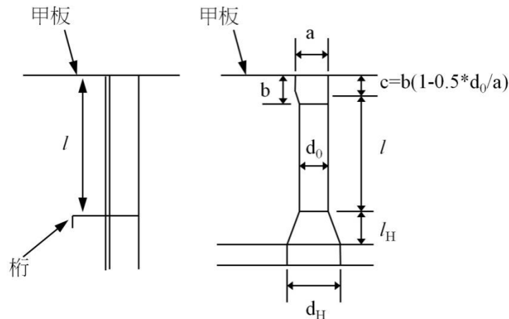
圖 II 16-1 l 的量測
