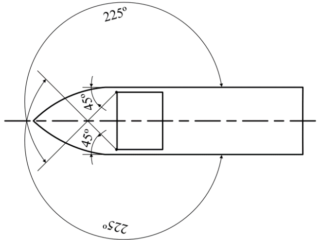
圖 III 6-3 每一駕駛橋艙兩翼之水平視野
