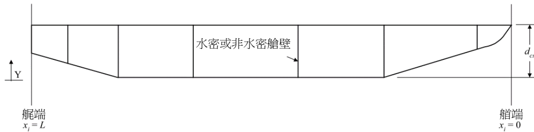
圖 III A2-1 橫跨甲板中心線剖面之典型幾何形狀
