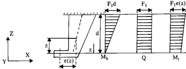
圖 II 2-3 舵掛角負荷
