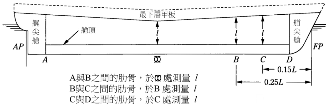
圖 II 6-1 艙肋骨的 l 量測點
