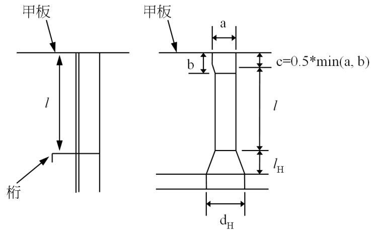
圖 II 14-3 l 的量測
