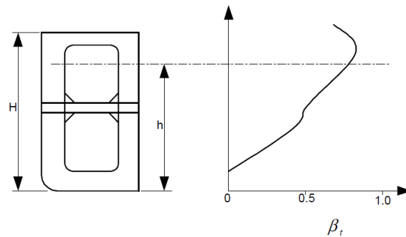
圖 II 33-2 大肋骨係數
