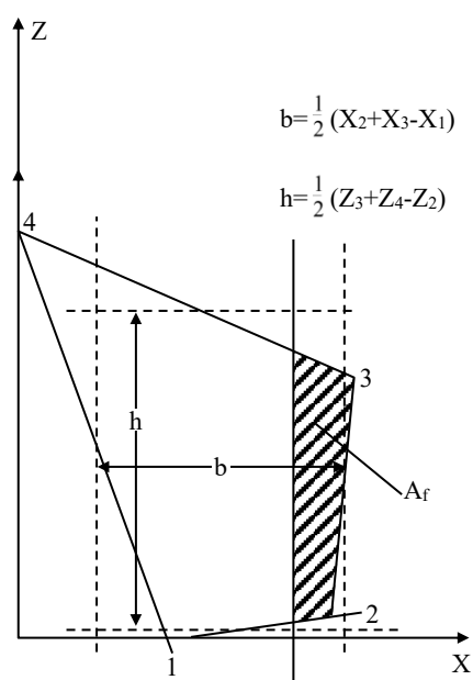
圖 II 24-3 完整舵葉
