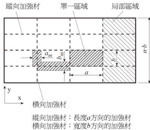
圖 II 17-3 嵌板的一般佈置
