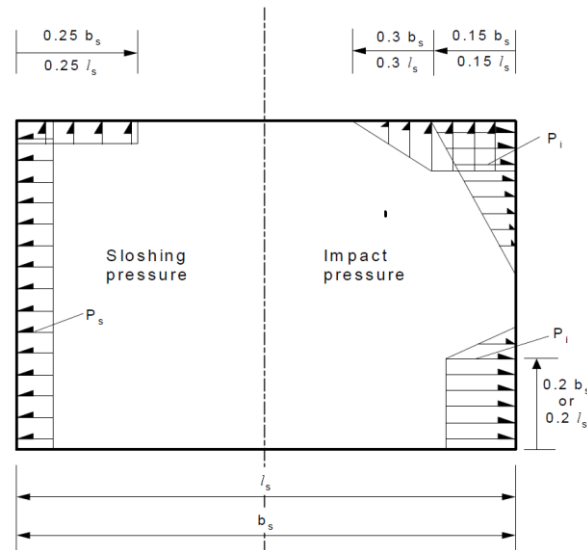
圖 II 33-3 壓力分佈
