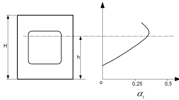
圖 II 33-1 制水艙壁係數
