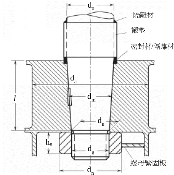
圖 II 24-7 帶鍵片錐形聯結器
