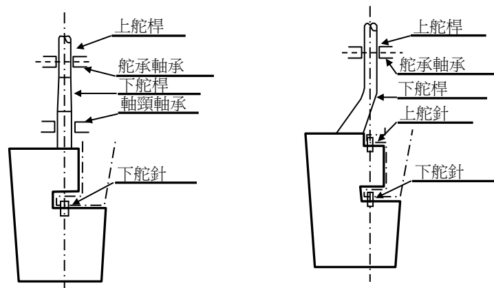
圖 II 24-2 舵掛角支撐型舵
