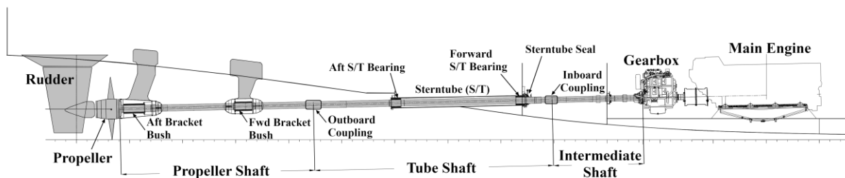
圖 I 2-1 典型的水潤滑軸系
