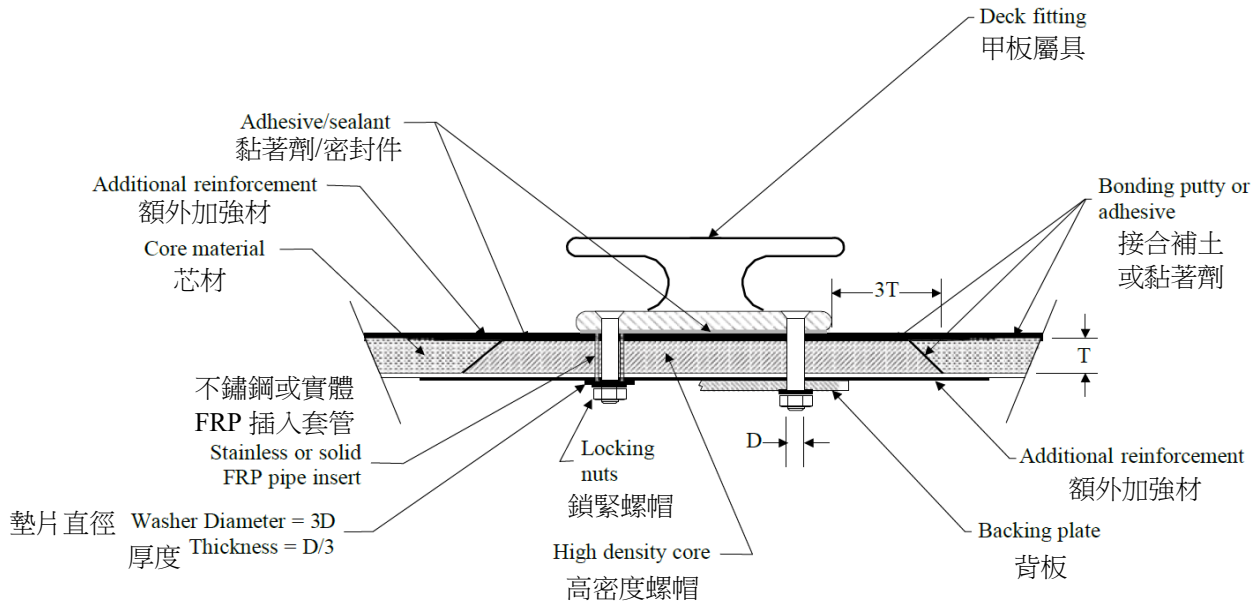
圖 III 2-26 甲板裝具
