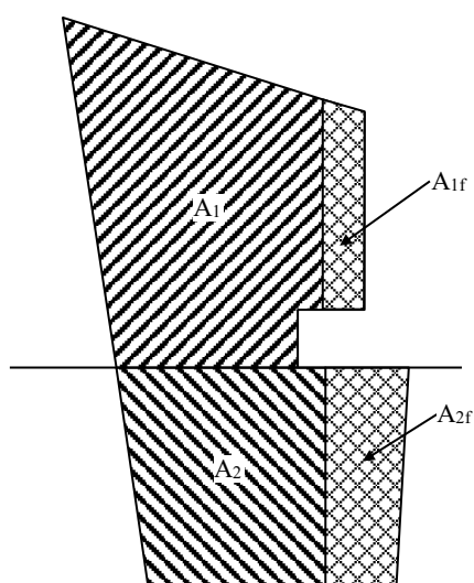
圖 II 24-4 缺角舵葉
