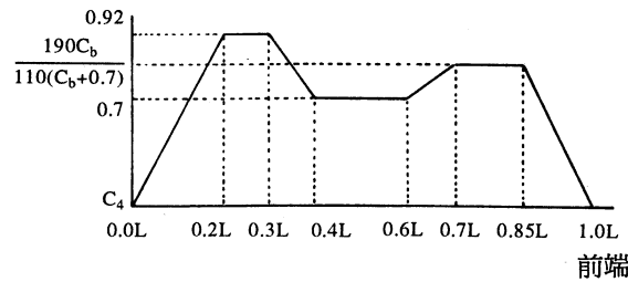
圖 II 3-5 分佈係數 C_4
