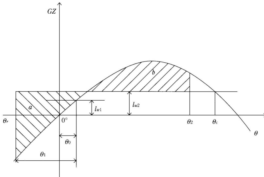
圖 II 30-2 穩度及風力傾側力臂曲線(強風與橫搖之穩度準則)
