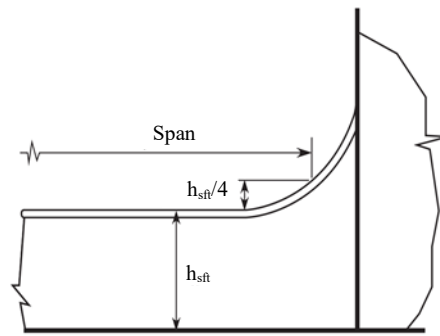
圖 II 1-4 沿著腋板邊緣具有連續面板之局部支撐構件的有效彎曲跨距
