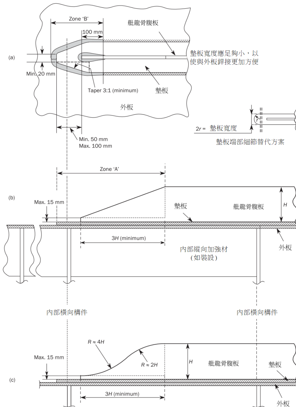
圖 II 1-9 舢龍骨端部設計
