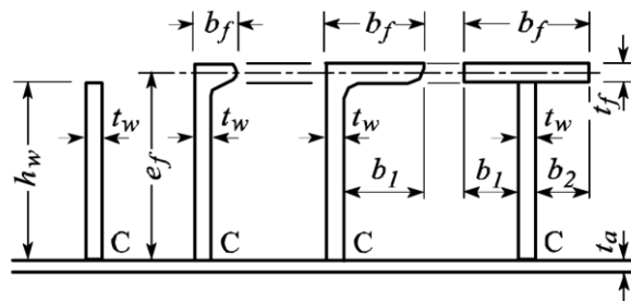
圖 II 17-6 加強材尺寸
