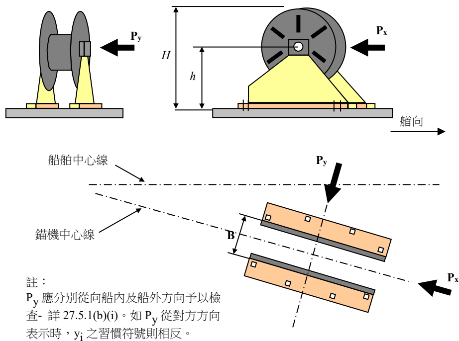
圖 II 27-3 力與重量之方向
