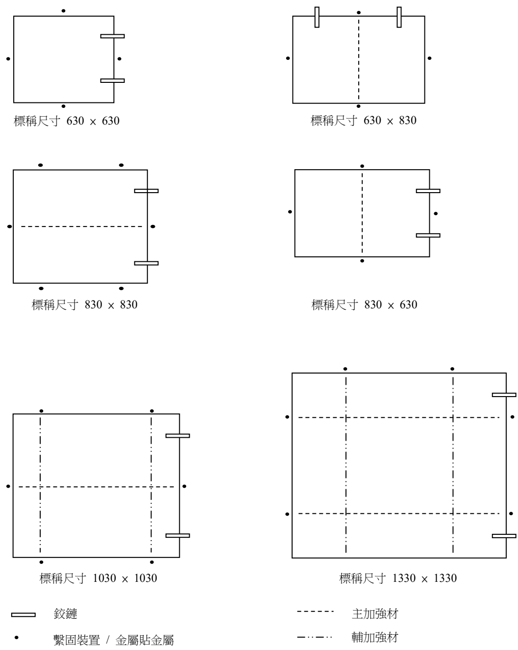
圖 II 27-1 加強材之佈置
