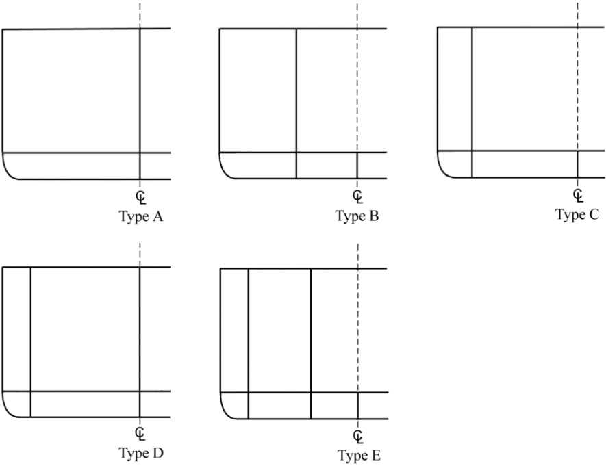
圖 II 3-6 有縱向隔艙壁之船舶的類型
