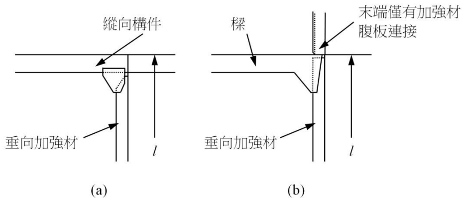
圖 II 14-1 端部連接型式
