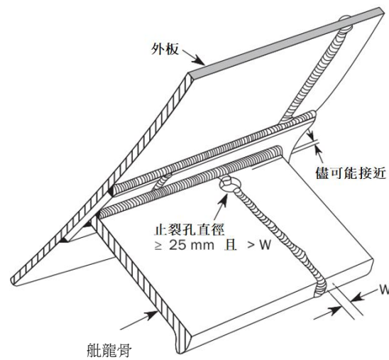
圖 II 1-8 舳龍骨構造
