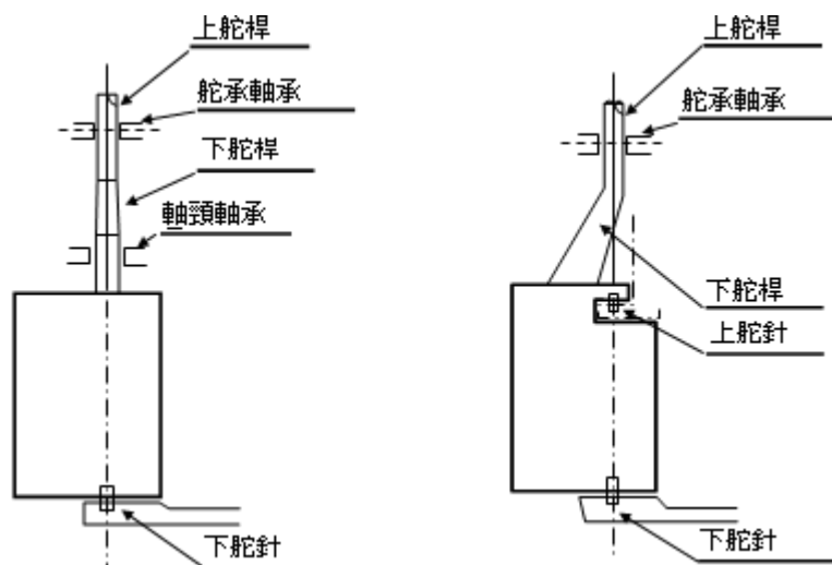
圖 II 24-1 舵跟材支撐型舵
