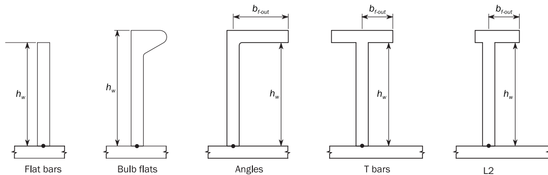
Figure 1 : Stiffener scantling parameters
