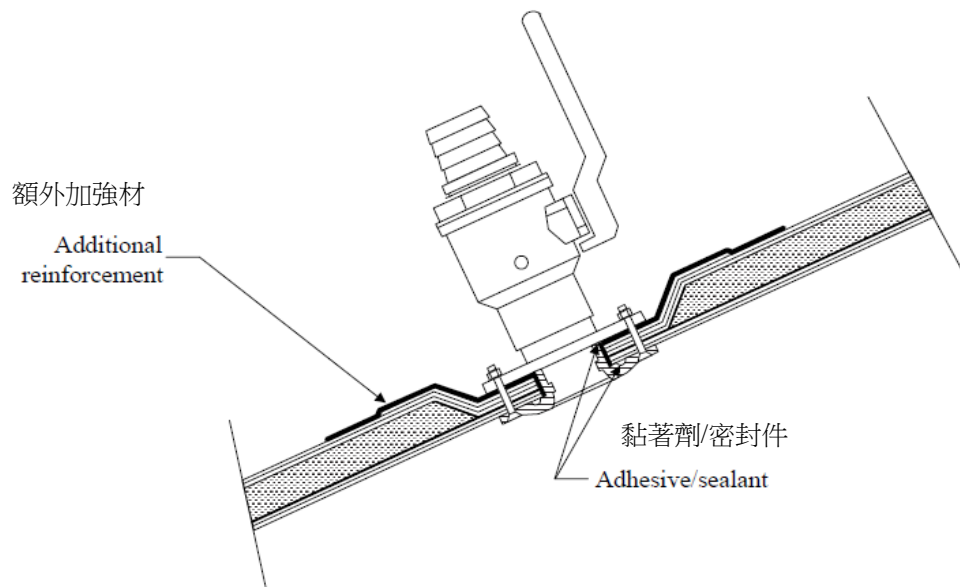
圖 III 2-27
