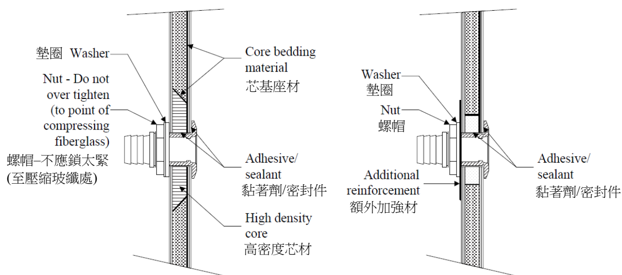
圖 III 2-28 穿過船殼貫穿件-三明治積層
