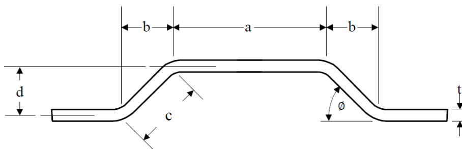
圖 III 2-15 波形艙壁
