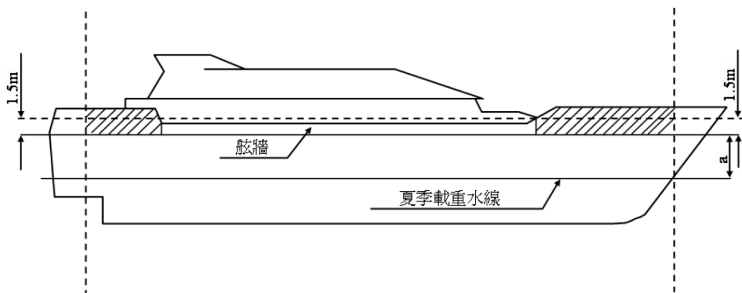
圖 III 5-1
