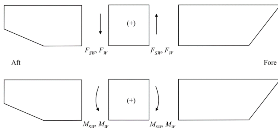
圖 III 2-1 正負符號
