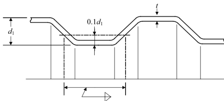
圖 III 2-16 波形艙壁端部連接
