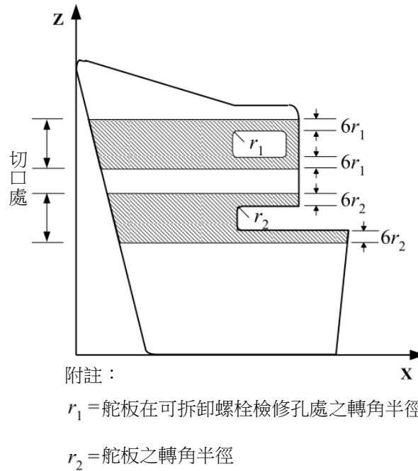
圖 III 2-48
