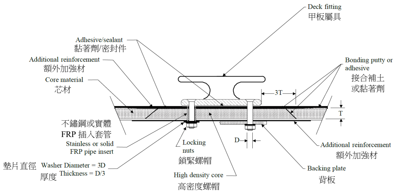
圖 III 2-26
