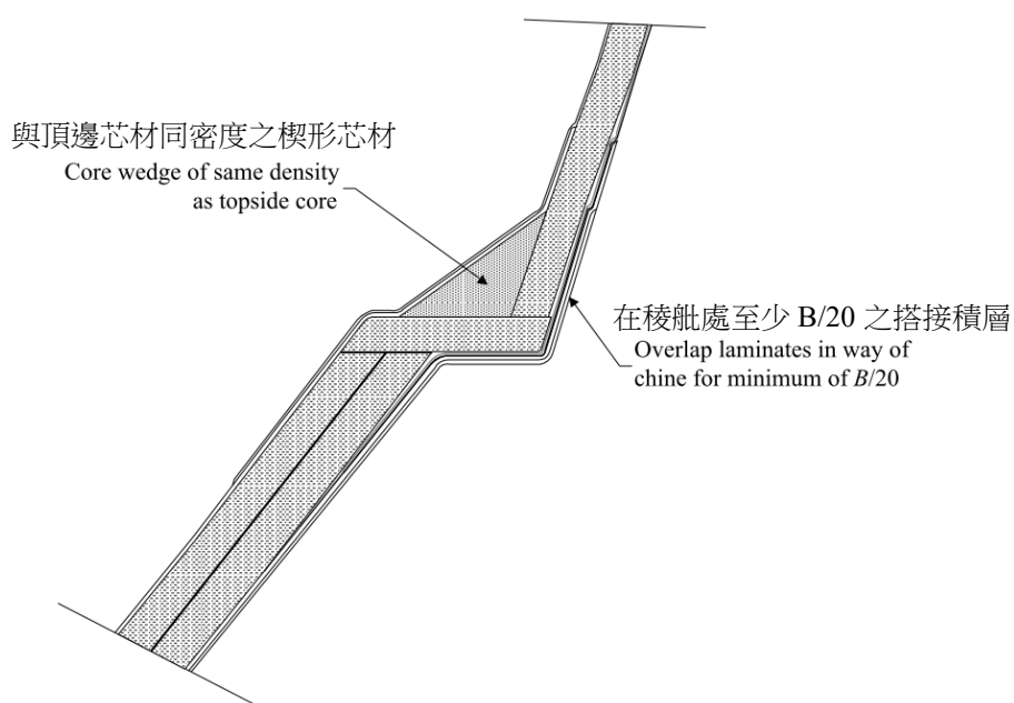
圖 III 2-36 階梯式稜艫-楔形發泡材選擇
