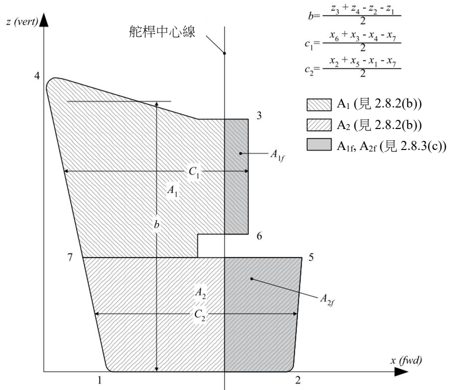
圖 III 2-40 缺角舵葉
