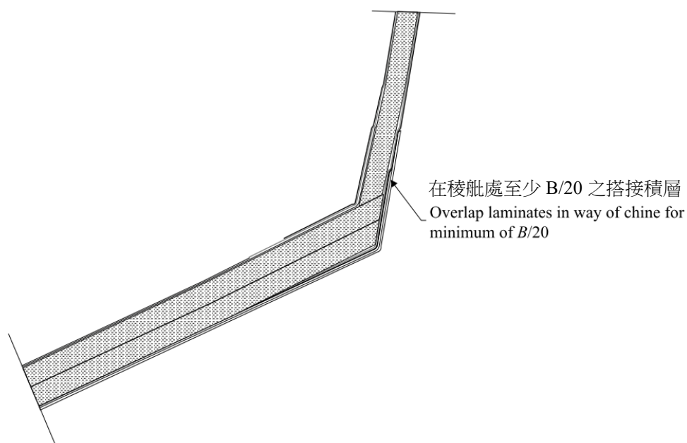
圖 III 2-35 稜艫或艫橫板-三明治構造
