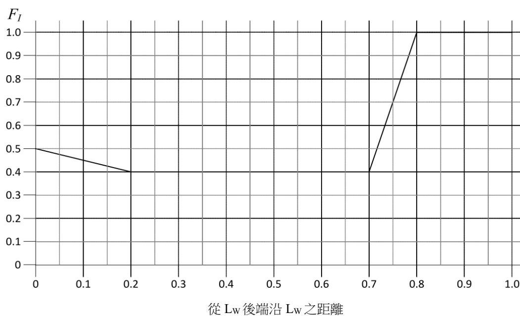
圖 III 2-10 濕面積分配係數 F_l
