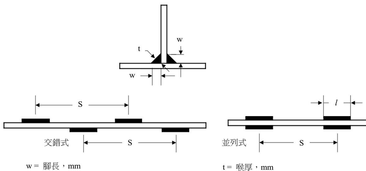
圖 II 2-5 斷續填角鉚
