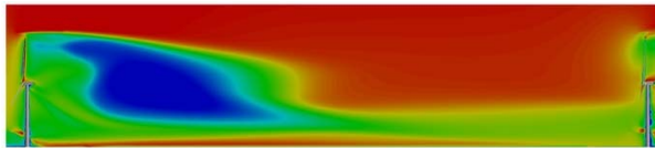
圖 6 前後排列風機間流場( \alpha_s = 12^\circ )
