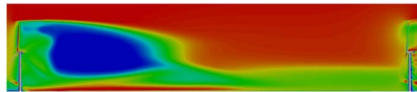
圖 7 前後排列風機間流場( \alpha_s = 15^\circ )
