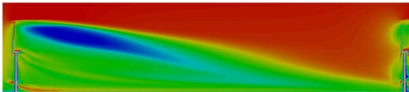
圖 4 前後排列風機間流場( \alpha_s = 6^\circ )
