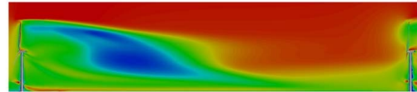
圖 5 前後排列風機間流場( \alpha_s = 9^\circ )
