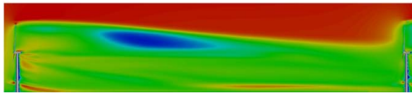
圖 2 前後排列風機間流場( \alpha_s = 0^\circ )
