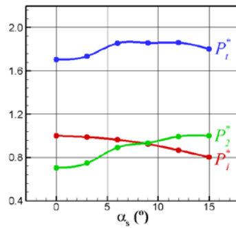
圖 8 前後排列風機無因次功率輸出
