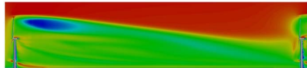
圖 3 前後排列風機間流場( \alpha_s = 3^\circ )
