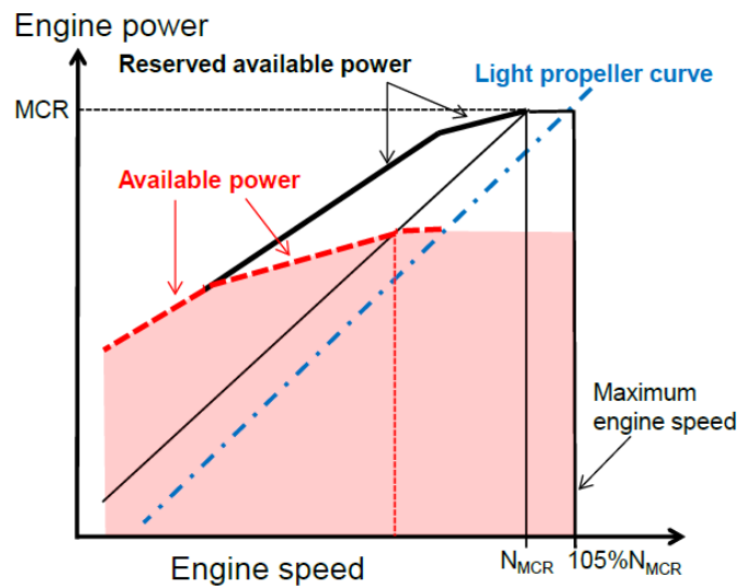
圖 2、Mechanical EPL 之主機負荷圖
