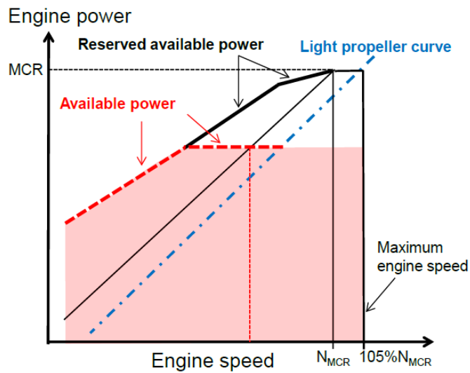
圖 1、ShaPoLi or electronic EPL 之主機負荷圖
